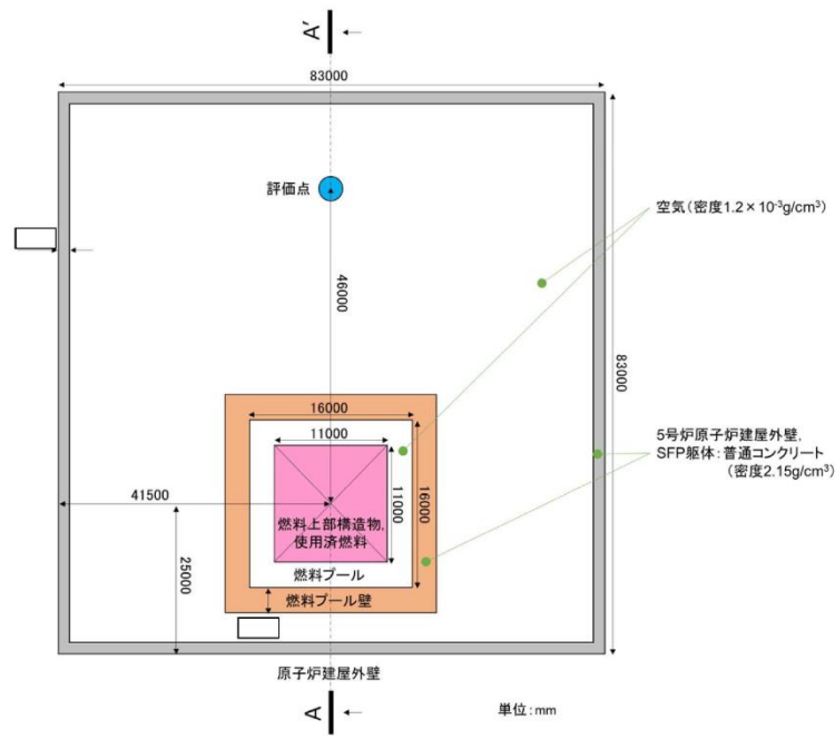
図添 1-12-1 線源モデル (使用済燃料・燃料上部構造物) (平面図)
