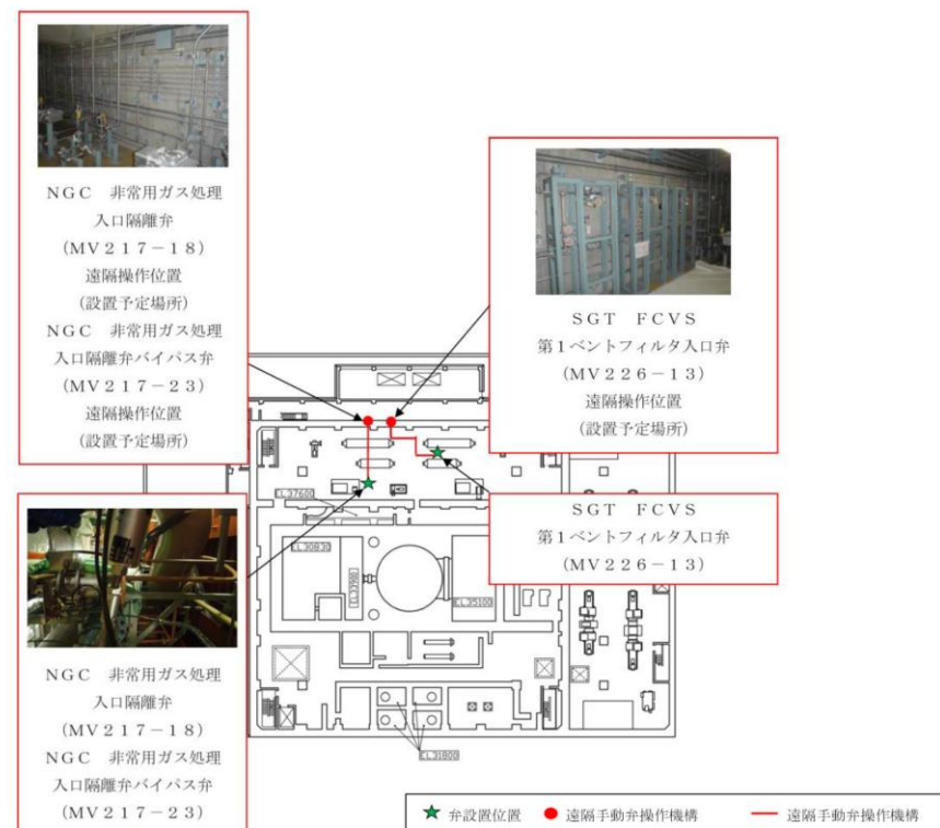
原子炉建物3階 【EL. 34800】
