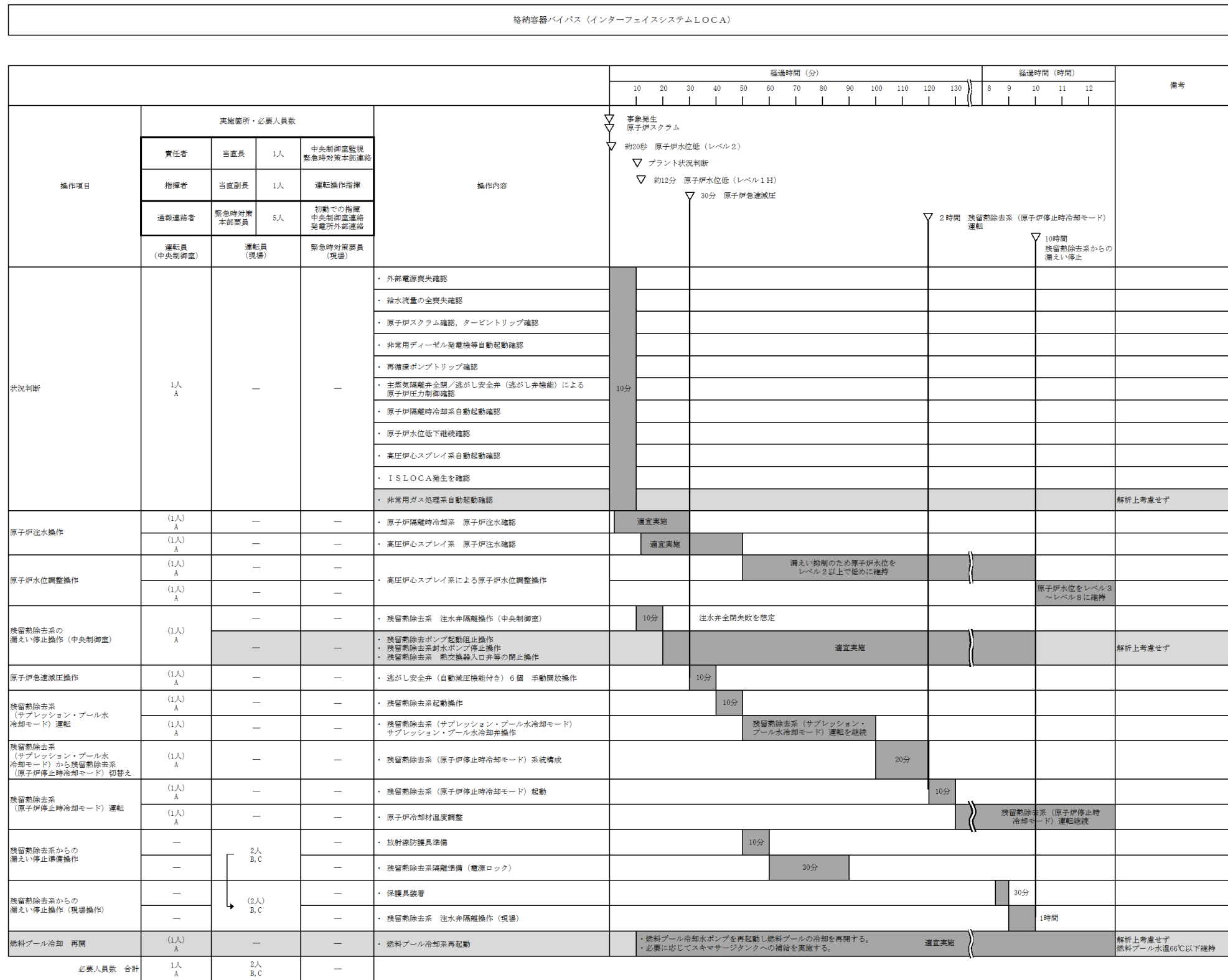
第 2.7.1-3 図 「格納容器バイパス (ISLOCA)」 の作業と所要時間
