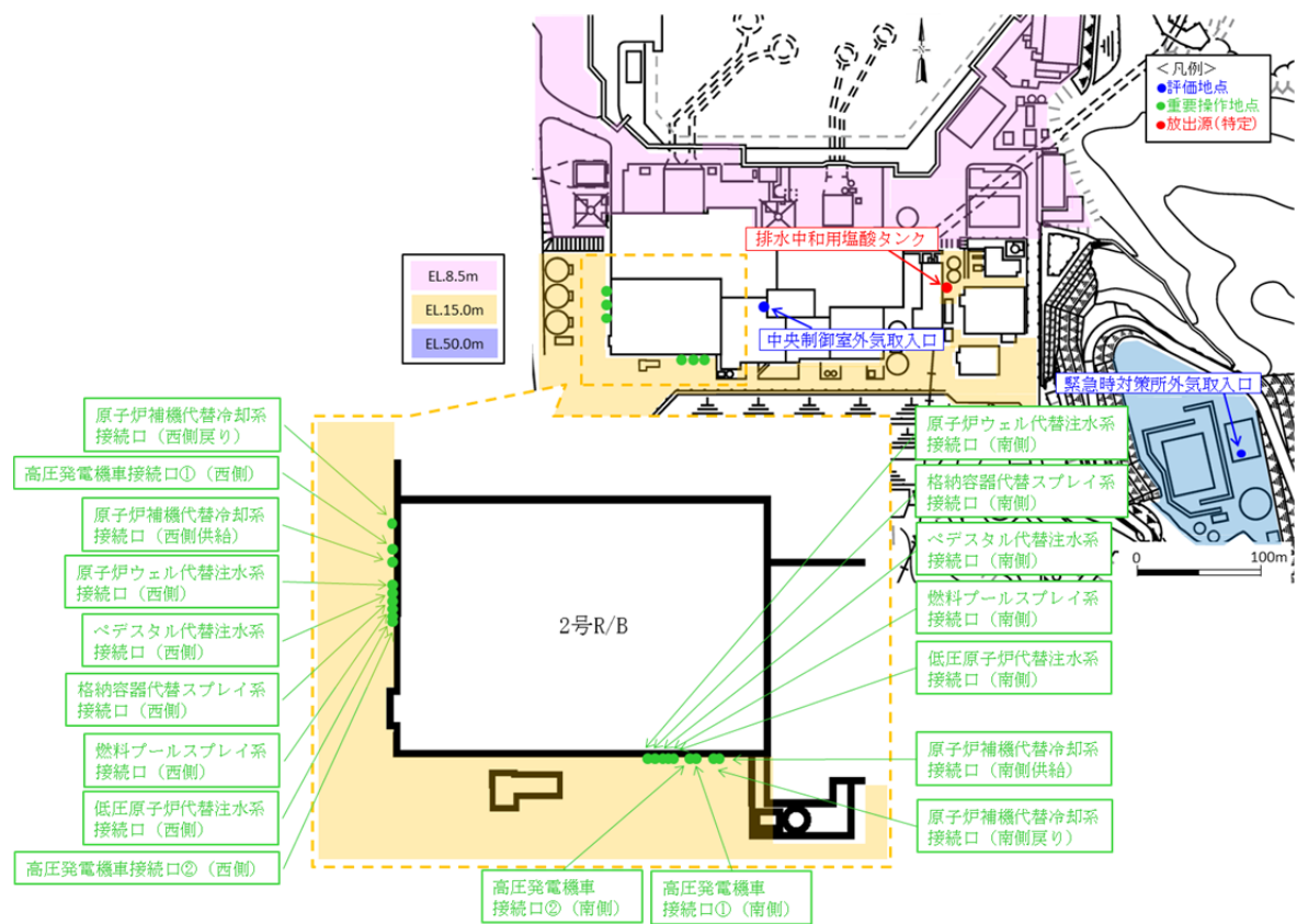
第3.1.1-4-1図 平面図
