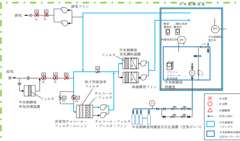
図 2.4-14 中央制御室換気系及び中央制御室待避室正圧化装置の概要図 (重大事故発生時, プルーフ通過中)
