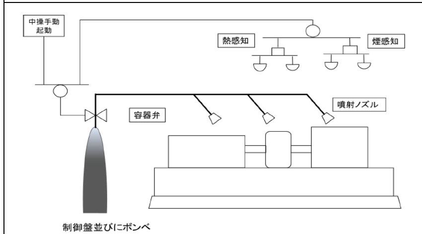
第 3.3 図：油内包機器に対する局所固定式消火設備概要図
