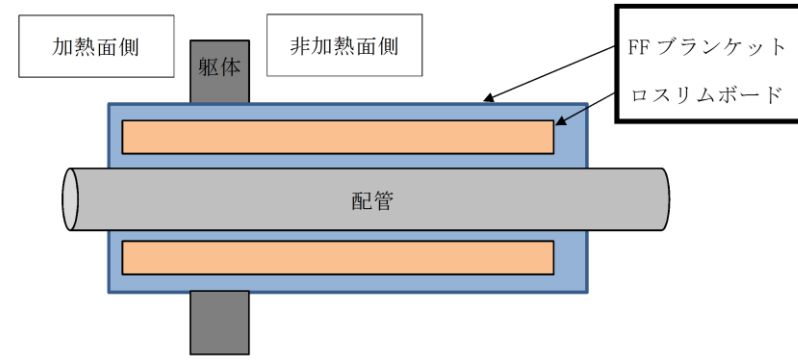
第1図 試験体概要
