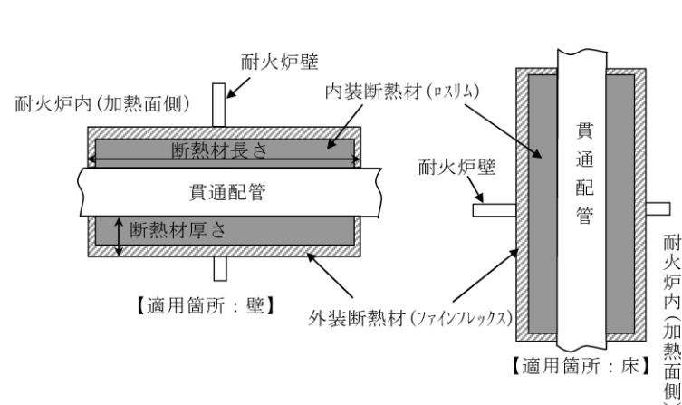
第4-1図 断熱材取付部の耐火試験体
