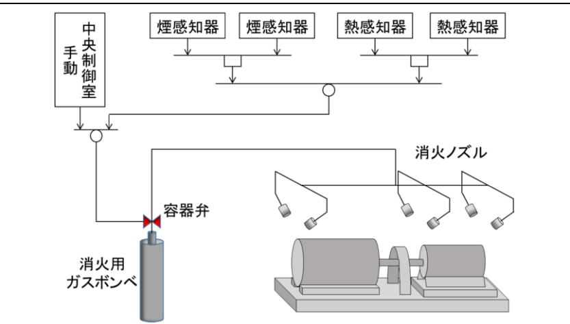
第 3 図 固定式のハロゲン化物自動消火設備(局所) (ハロン 1301) の概要
