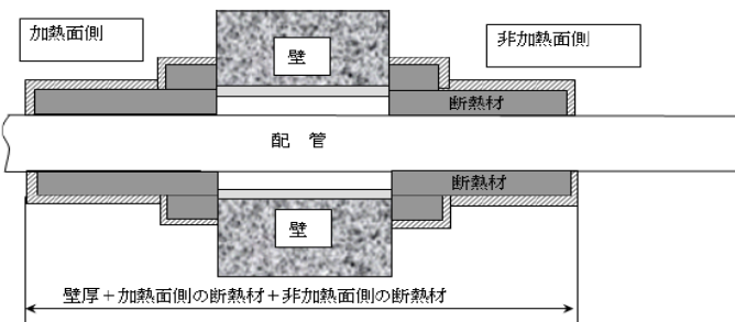
図3 耐火対策イメージ
