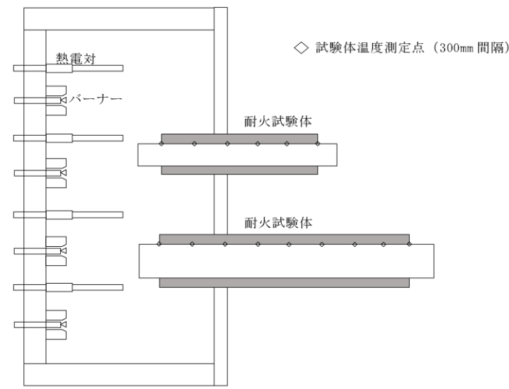
第 4-2 図 耐火試験炉
