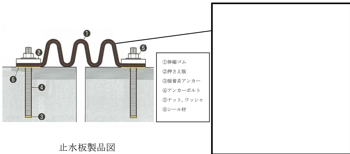
図1 止水板の概要
