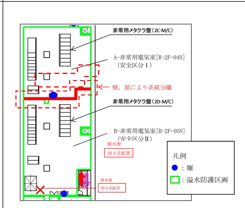
図5-12 非常用電気室の消火系配管の被水影響評価において溢水防護対象設備の多重化により同時に機能喪失しないと評価した例
