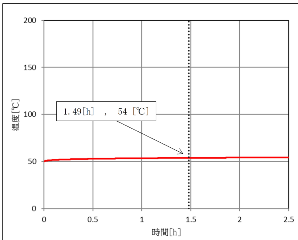
第2-4図 外壁面温度推移 (空中給油機等)
