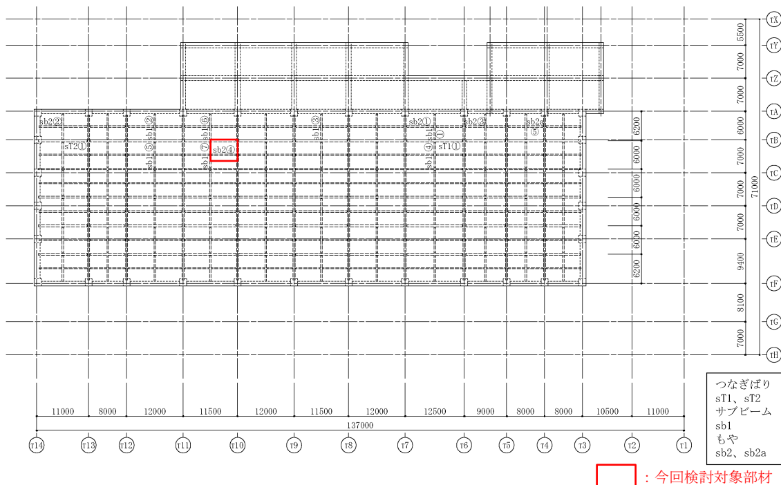
第 3-3 図 部材位置図（トラス二次部材：母屋）
