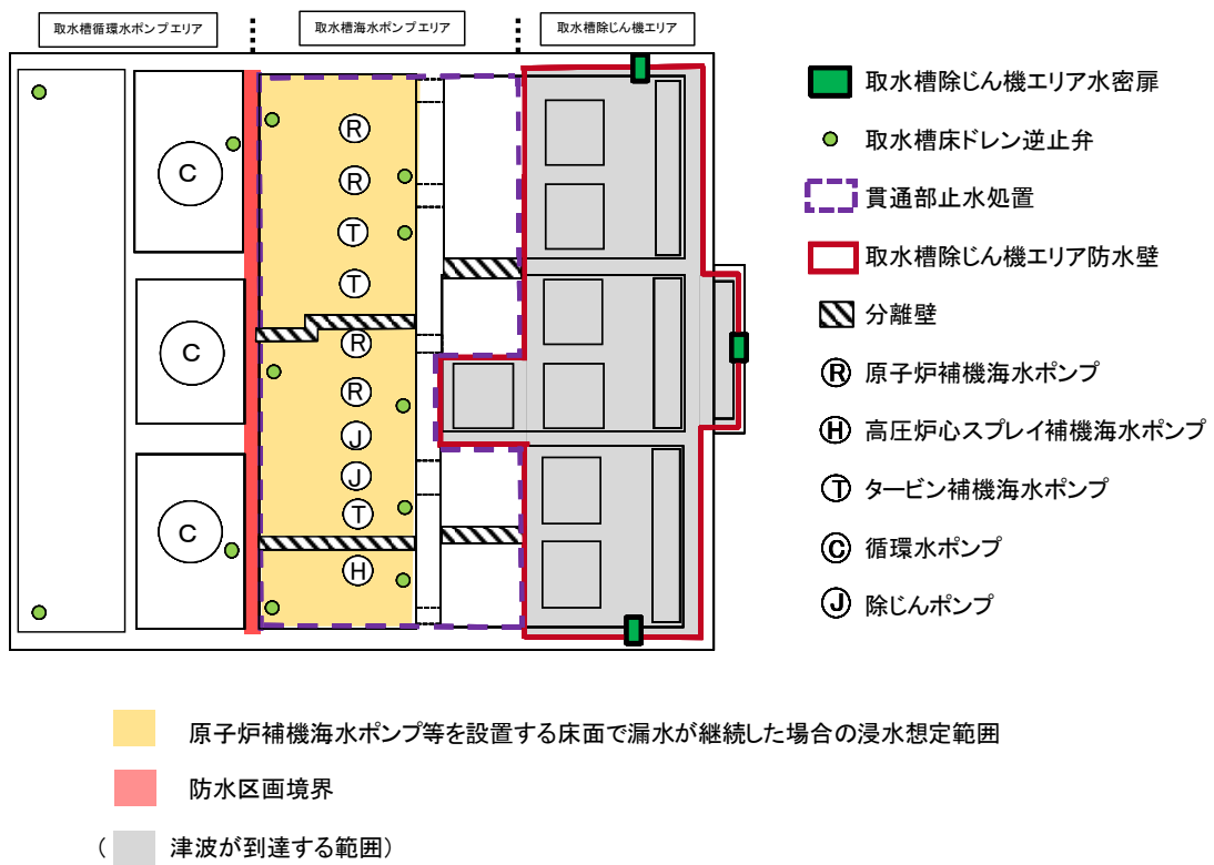
第 1.5-12 図(2) 浸水想定範囲（取水槽海水ポンプエリア）に対する 防水区画化範囲
