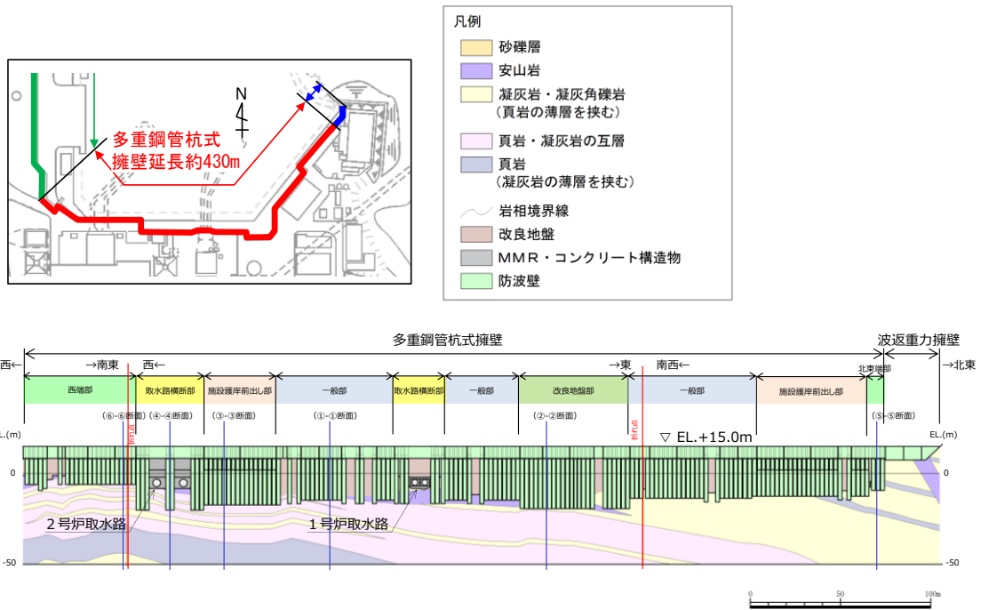
第 5-10 図 防波壁（多重鋼管杭式擁壁）の地質縦断面図
