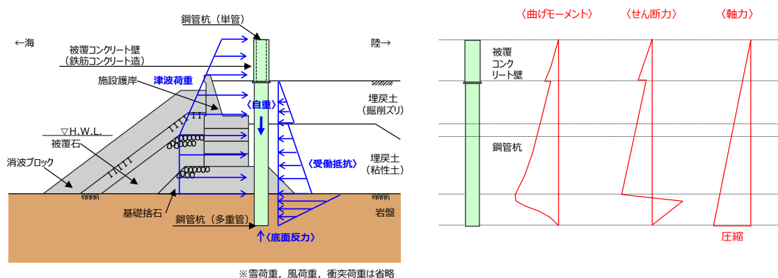
荷重図
