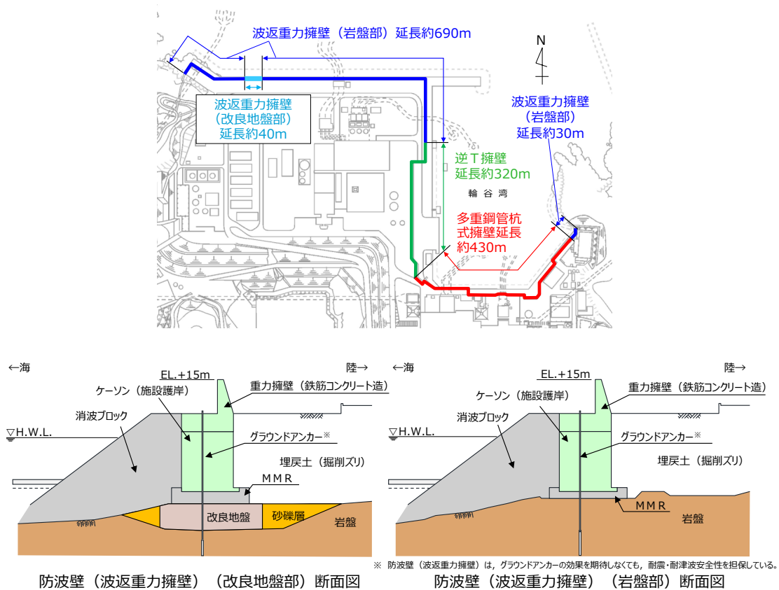
第7-1図 防波壁（波返重力擁壁）の構造概要図
