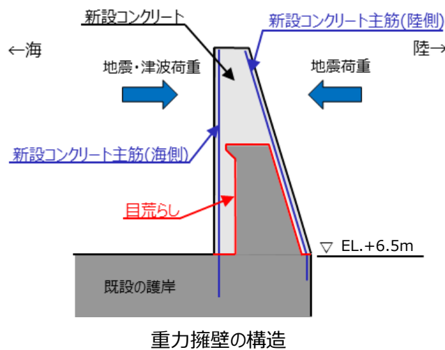
第7-36図 重力擁壁の構造図
