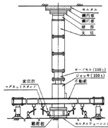
第6-31図 防波壁（逆T擁壁）平板載荷試験概要
