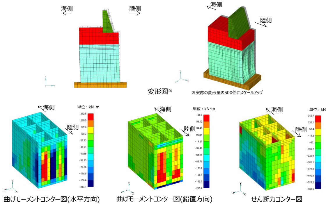
第10-5-13 図 3次元静的FEM解析結果（輪谷部）
