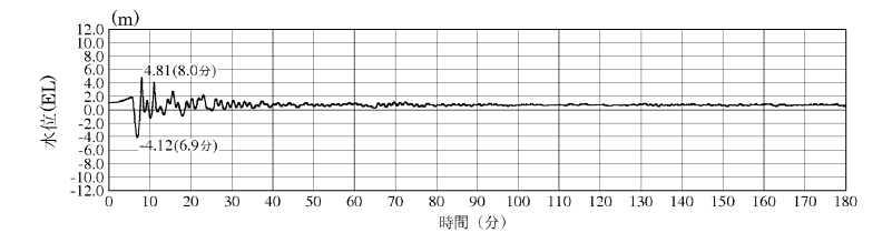
2号炉取水槽 (入力津波4, 防波堤無し)
