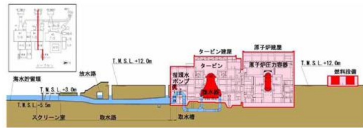
取水路断面
