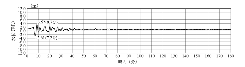
3号炉取水槽 (入力津波4, 防波堤有り)
