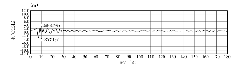
1号炉取水槽 (入力津波4, 防波堤有り)
