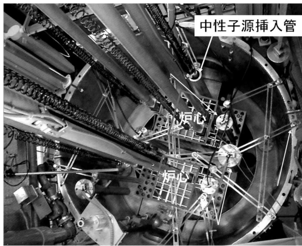
図 A-2 炉心内の中性子源挿入管
