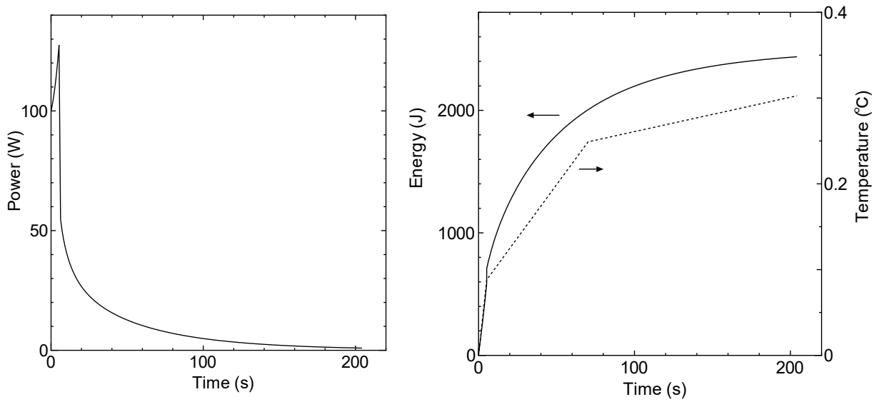
図 2-1 L5.5P-30(炉心高 30.8cm)炉心 出力変化 (左)、積算出力と温度変化 (右実線：出力、右点線：温度) (右図の横軸は制御棒挿入時からの経過時間)
