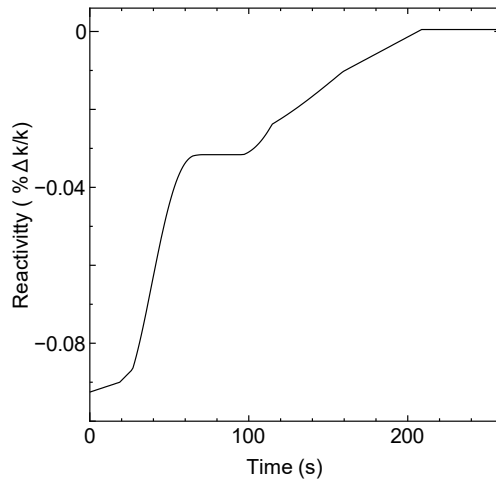
図 7-11 L2-P30(最小) 反応度変化 (中心架台上昇は 208 秒まで)
