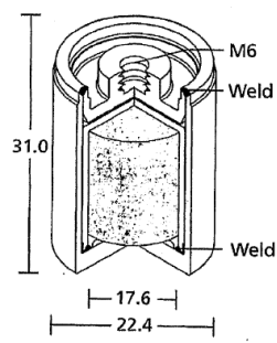
図 A-1 Am-Be 中性子源の構造
