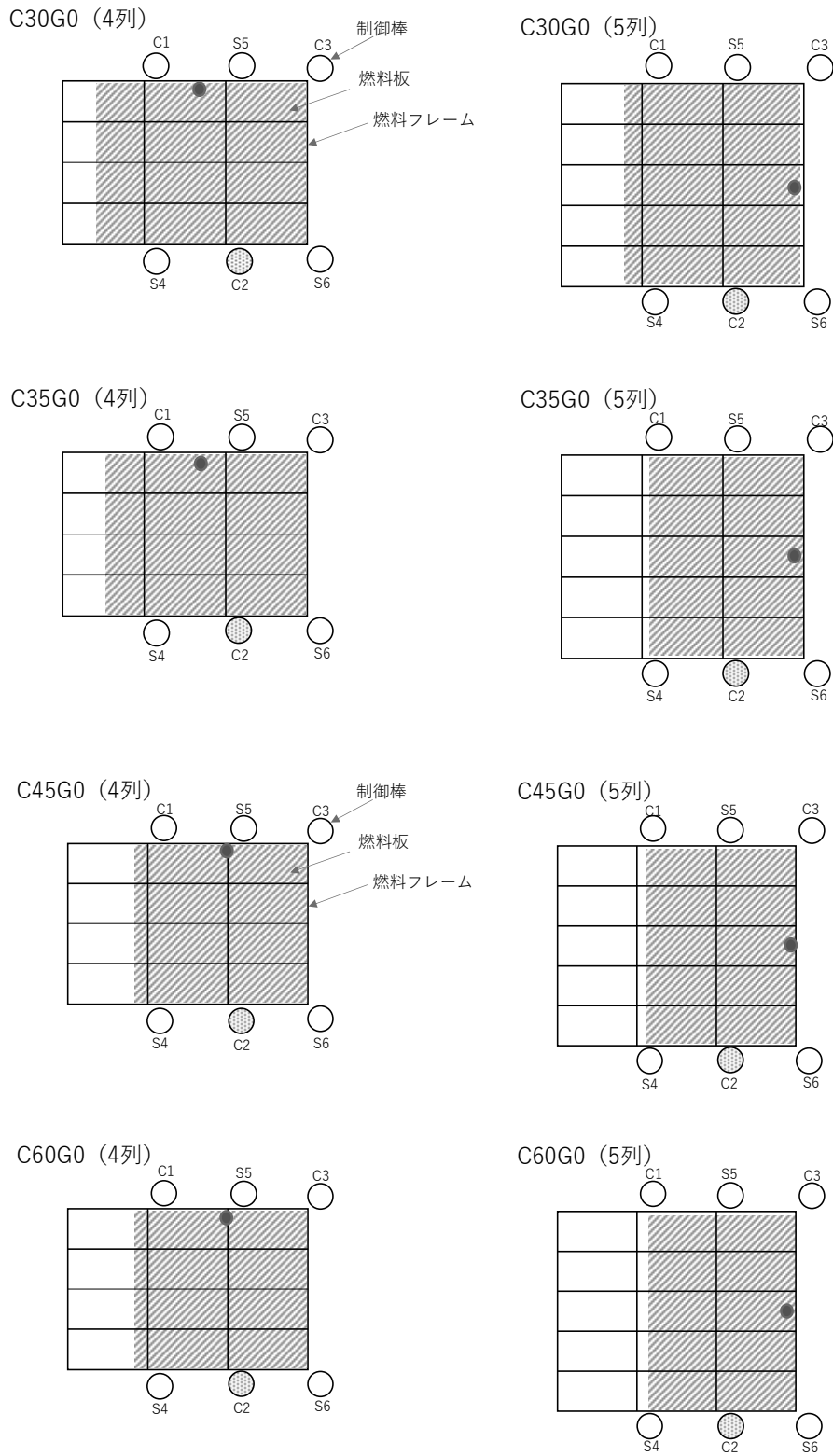
図 A-5 軽水減速炉心の炉心配置図 (1) (炉心内丸印が出力分布が最大となる点)
