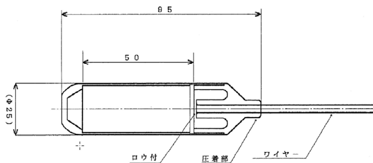
図A-4 中性子源取り付けカプセル
