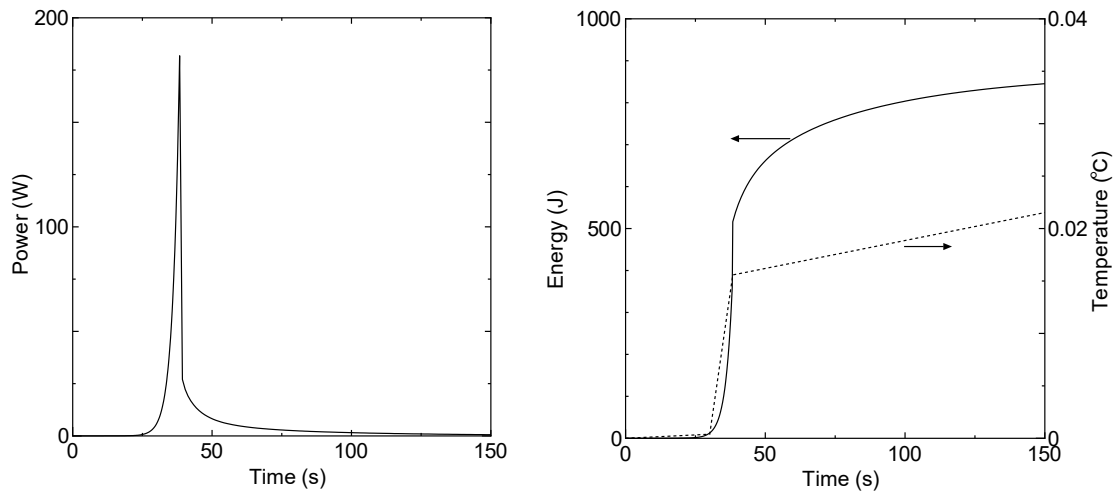
図1-2 C45G(2H 2 O) 4列炉心 出力変化(左)、積算出力と温度変化(右実線:出力、右点線:温度) 原子炉起動時における制御棒の異常な引抜き(ケースA)
