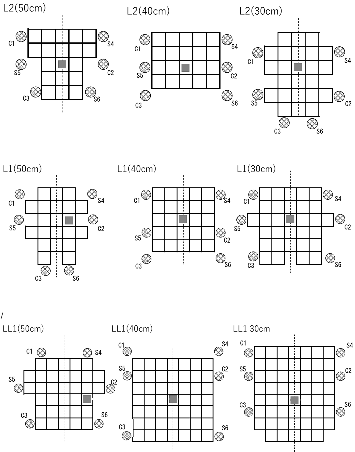
図 8 - 3 炉心配置図 (L2P、L1P、LL1P) (■の記号をつけた燃料体が核分裂の積分値が最大となる燃料体)
