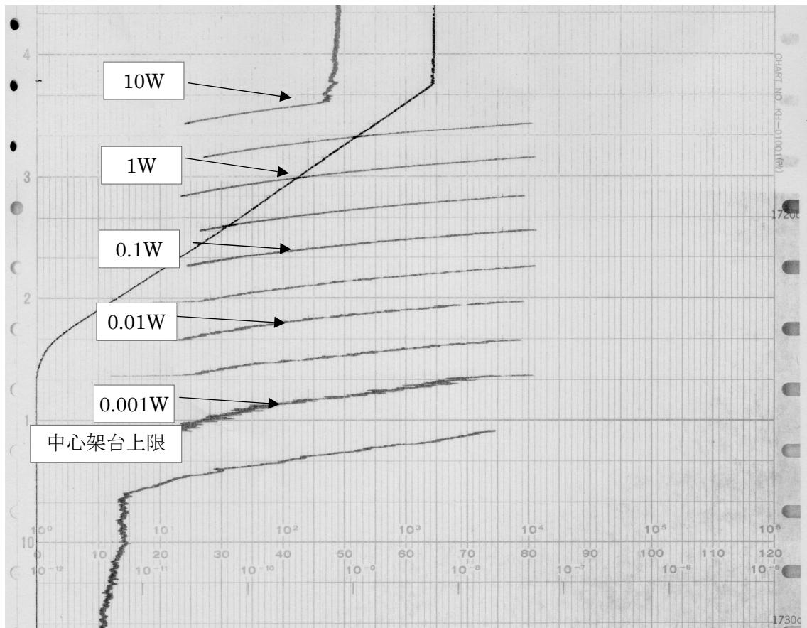
図 線型出力計 指示値 (チャート紙) (図の下方から上方へ時間が経過する。 一番上で出力が一定となっているところが出力約 10W のところ)
