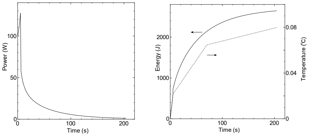
図 2-2 C45G(2H 2 O) 4 列炉心 出力変化 (左)、積算出力と温度変化 (右実線：出力、右点線：温度) (右図の横軸は制御棒挿入時からの経過時間)
