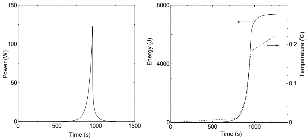
図 3-4 C45G(2H 2 O) 4 列炉心 出力変化
