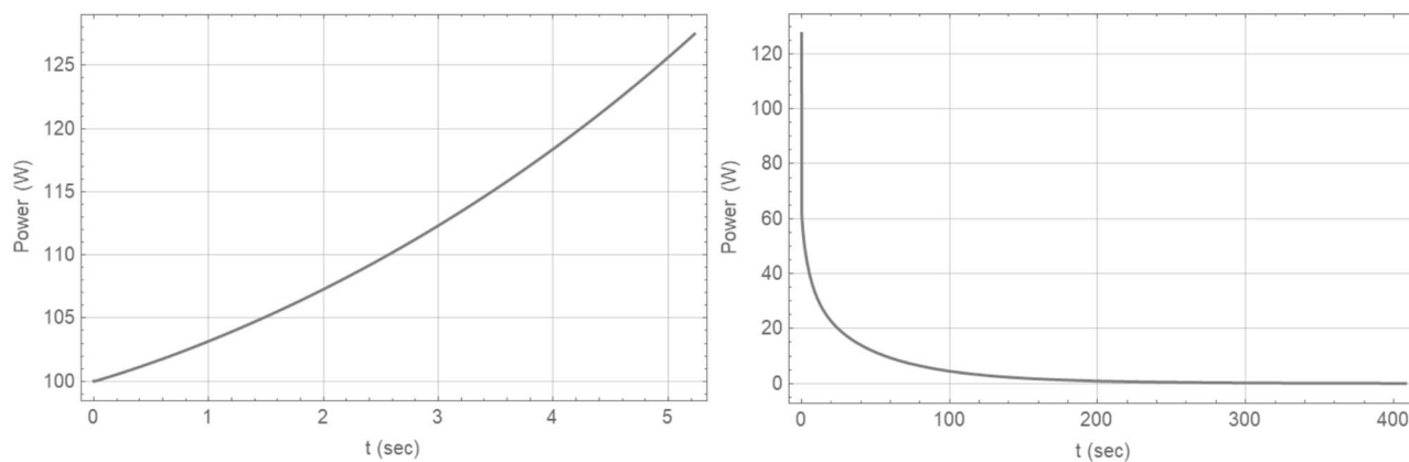
図 2-1 L5.5P-30(炉心高 30.8cm)炉心 出力変化 出力運転中の制御棒の異常な引抜き(ケース A) (右図の横軸は制御棒挿入時からの経過時間)
