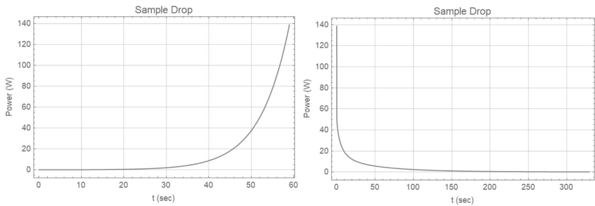
図 3-1 L5.5P-30 炉心 出力変化 (左 : スクラム前、右 : スクラム後) 実験物の異常等による反応度の付加 (ケース A ステップ状反応度添加)
