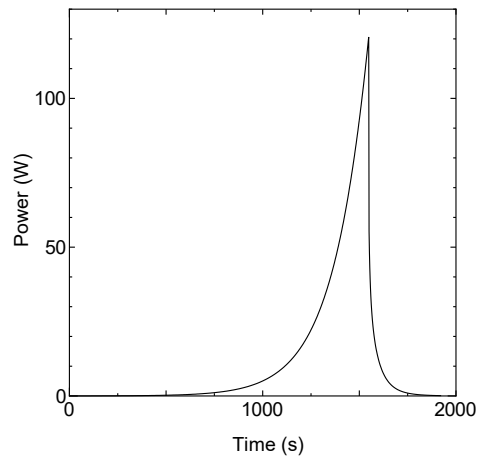
図 1 - 4 C45G(2H 2 O) 4 列炉心 出力変化 原子炉起動時における制御棒の異常な引抜き(ケース B)
