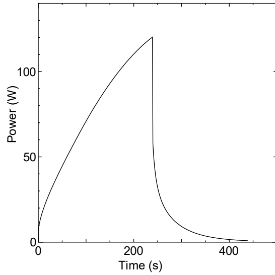
図 5-1 L5.5P-30 炉心 出力変化
