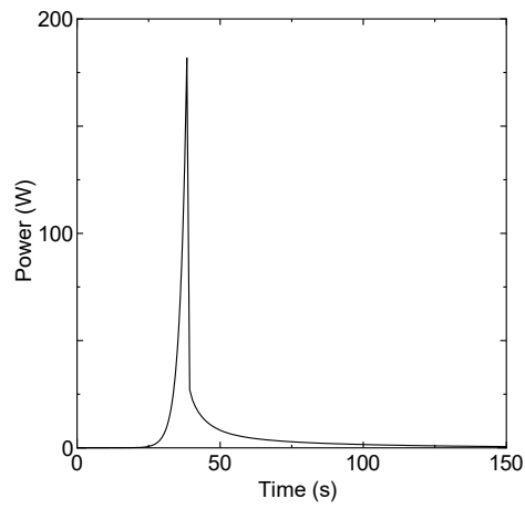
図 1 - 2 C45G(2H 2 O) 4 列炉心 出力変化 原子炉起動時における制御棒の異常な引抜き(ケース A)
