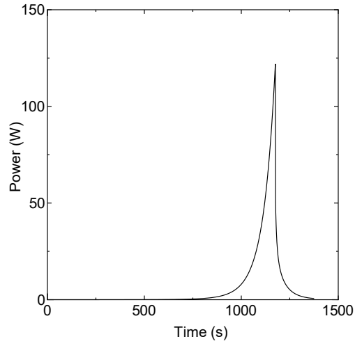
図 3-3 L5.5P-30 炉心 出力変化 実験物の異常等による反応度の付加 (ケース B ランプ状反応度添加)
