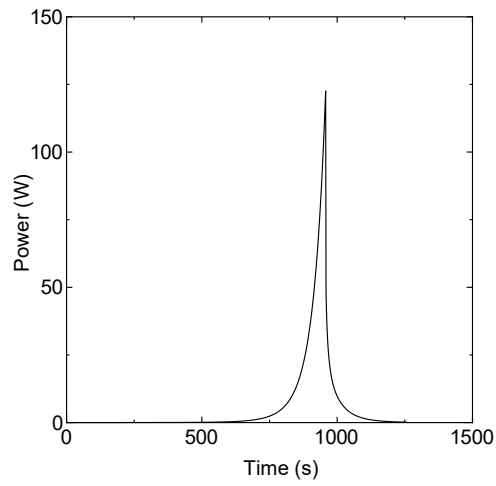
図 3-4 C45G(2H 2 O) 4 列炉心 出力変化 実験物の異常等による反応度の付加 (ケース B ランプ状反応度添加)
