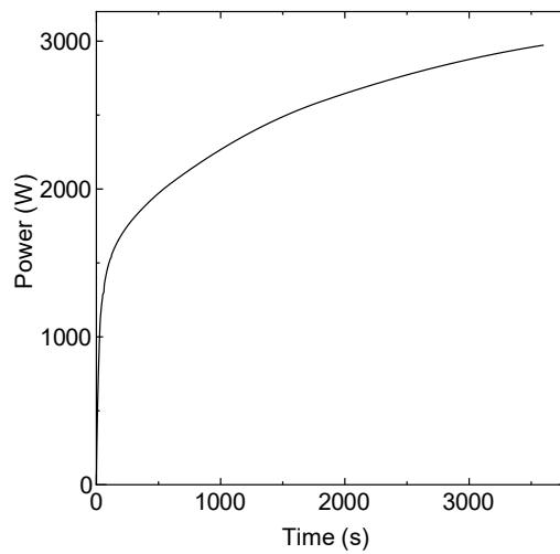
図 4-4 C45G(2H 2 O) 4 列炉心の積算出力 (中性子とガンマ線の積算)
