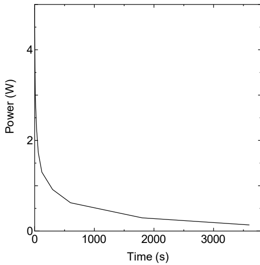
図 4-3 FP からの発熱 出力変化
