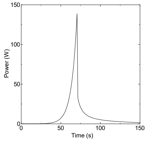
図 1 - 1 L5.5P-30(炉心高 30.8cm)炉心 出力変化 原子炉起動時における制御棒の異常な引抜き(ケース A)
