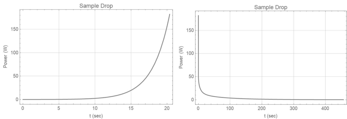
図 3-2 C45G(2H 2 O) 4 列炉心 出力変化 (左 : スクラム前、右 : スクラム後) 実験物の異常等による反応度の付加 (ケース A ステップ状反応度添加)
