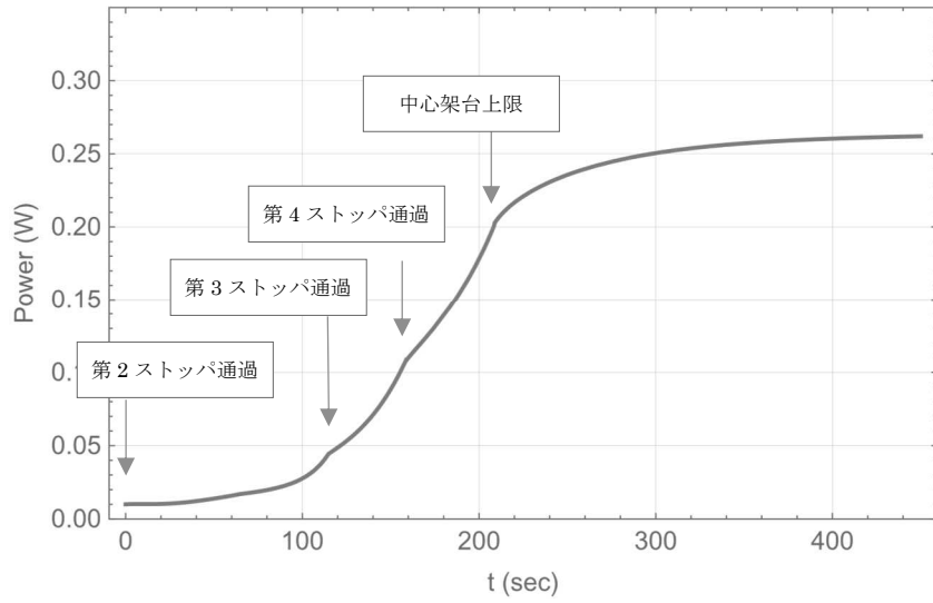
図 7-8 L5.5 (30cm) 炉心での通常運転時(燃料誤装荷無し) の中心架台上昇時の出力変化 (横軸、縦軸は図 7-6 と同じ)
