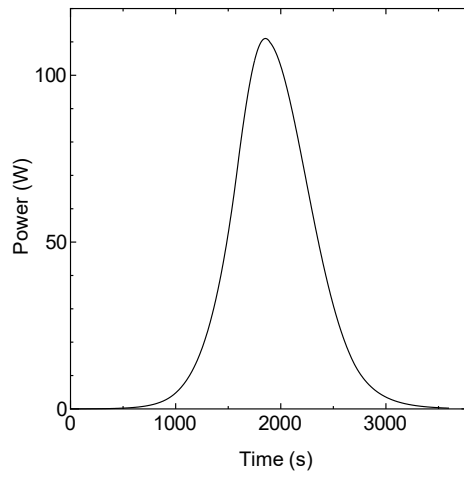
図 1 - 3 L4P-30 炉心 出力変化 原子炉起動時における制御棒の異常な引抜き(ケース B)
