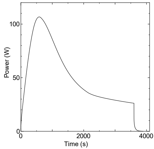
図 5-2 L1P-30 炉心 出力変化
