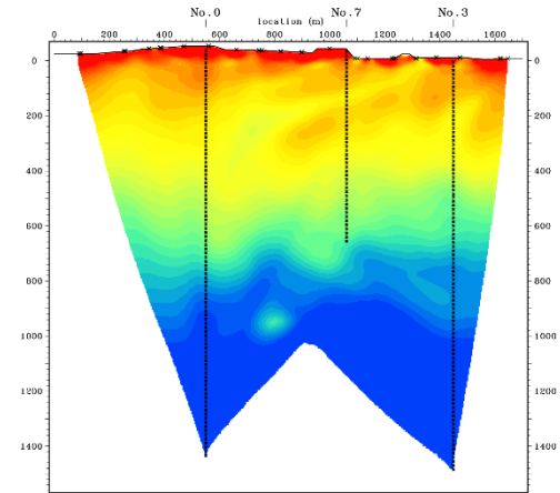
S波の初動解析結果（0-7-3測線）
