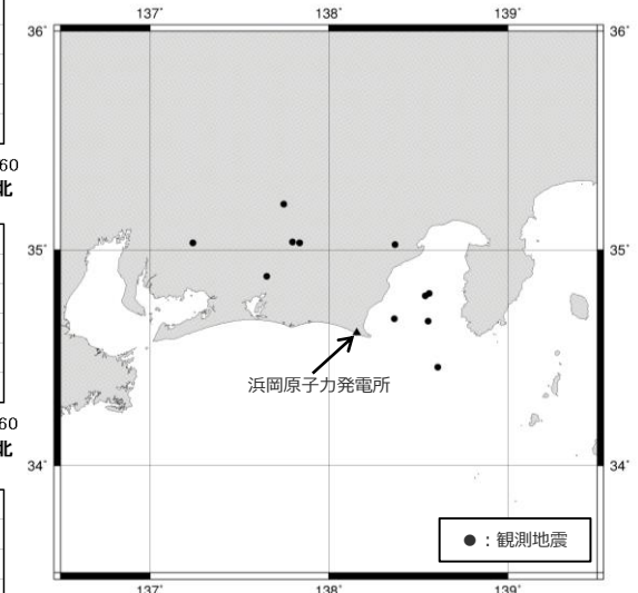
<各地震の震央分布>
