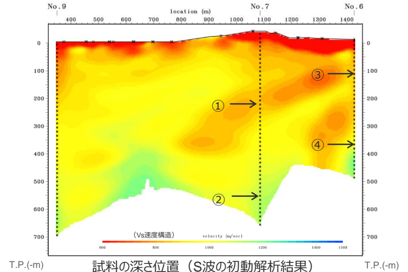
試料の深さ位置 (S波の初動解析結果)
