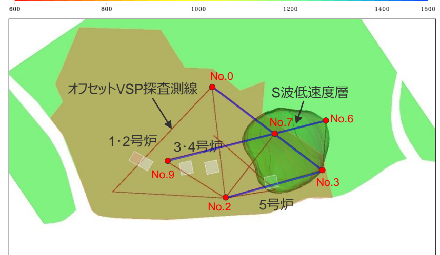
S波低速度層の分布 (平面図)
