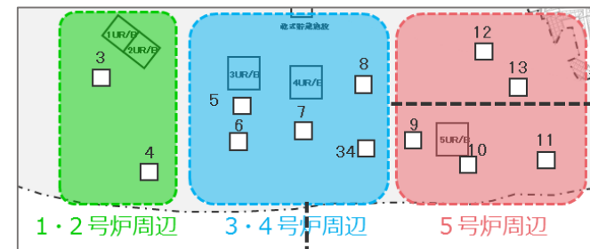
多点連続地震観測における地震計の配置
