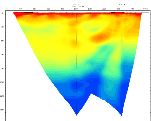
S波の初動解析結果（2-3測線）
