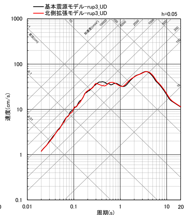
(UD方向)
