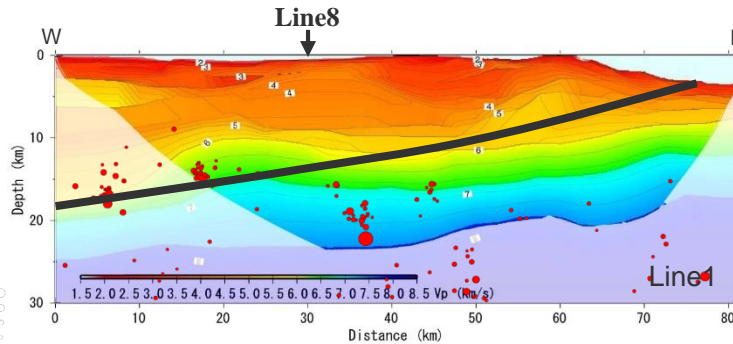
(断面図)
