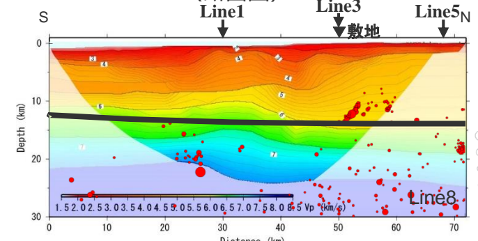
(断面図)
