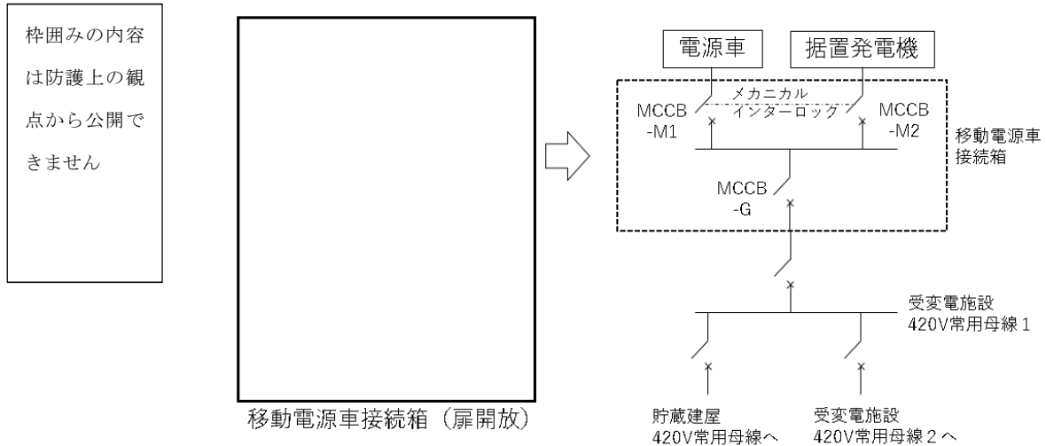
第 4-1 図 移動電源車接続箱と単線結線図
