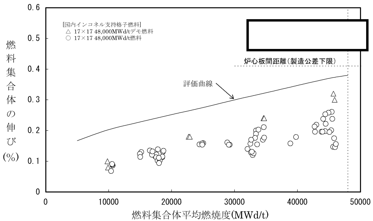
第3-13図 燃料集合体の伸び
