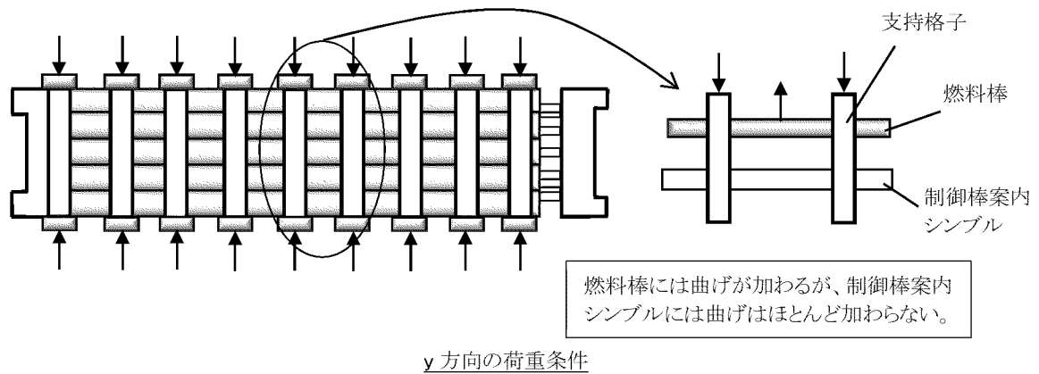
第 4-2 図 燃料集合体にかかる荷重
