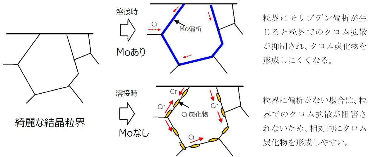
第1図 モリブデン添加による影響 (イメージ図)
