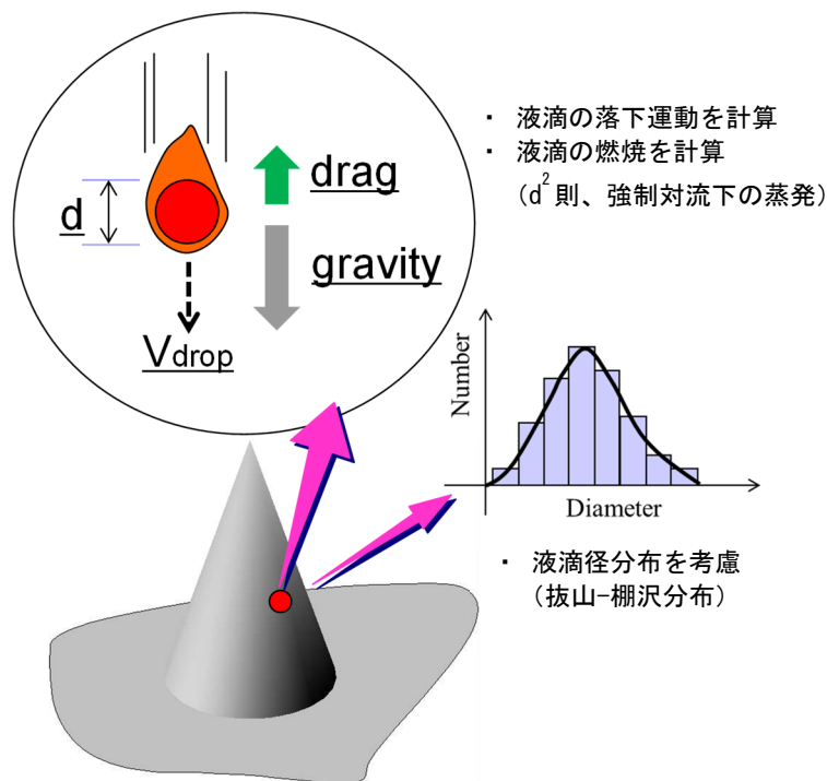
第4図 スpray燃焼モデルの概要
