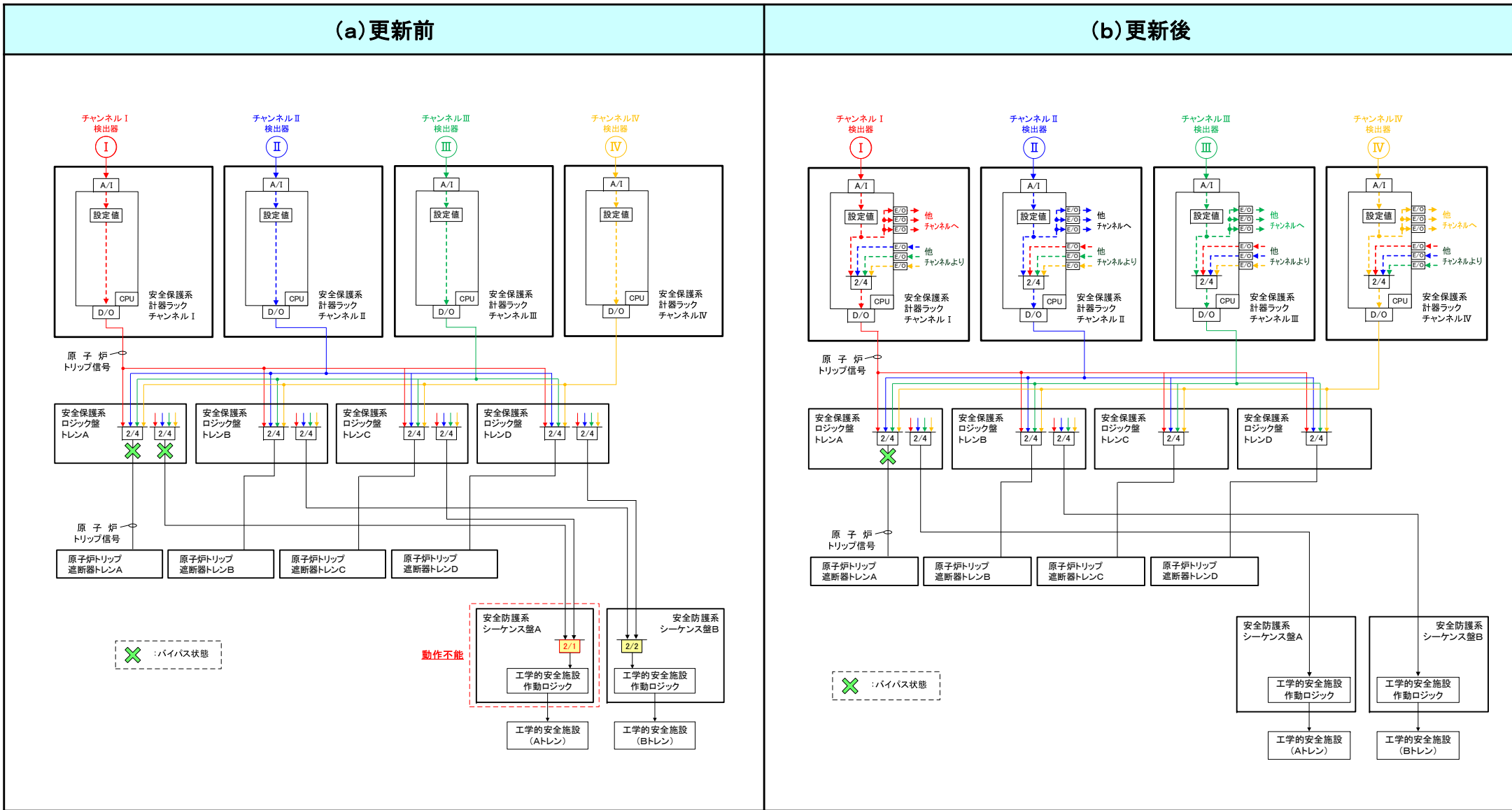
第13図 原子炉保護設備に係る定期点検（サーベイランス）時の状態
