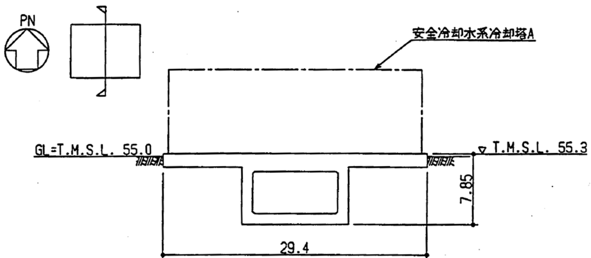
断面図 (NS方向)
