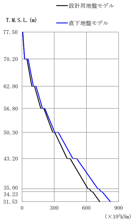
第 2.4.2.1-11 図 最大応答曲げモーメント (NS 方向 1.2 \times S_s - C1 (NSEW))
