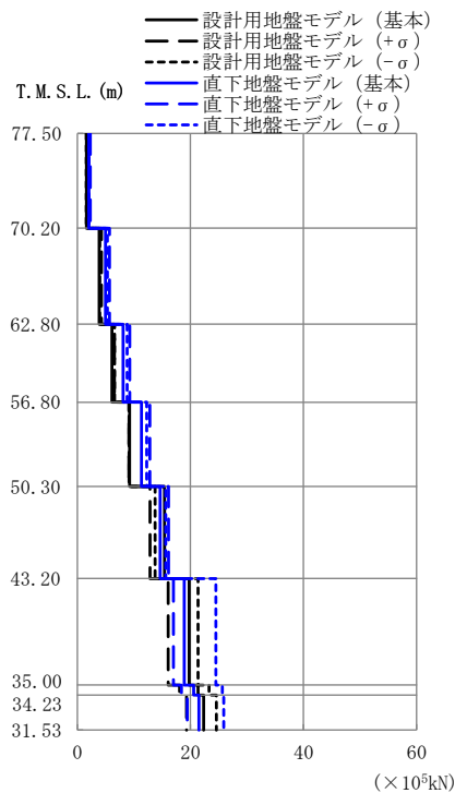
第 2.4.1.1-2 図 最大応答せん断力 (NS 方向 S s -A(H))
