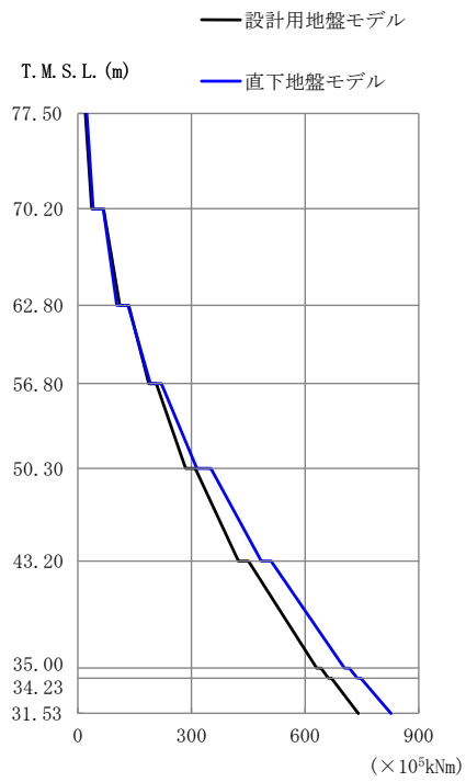
第 2.4.2.1-14 図 最大応答曲げモーメント (EW 方向 1.2 \times S_s-C1(NSEW) )
