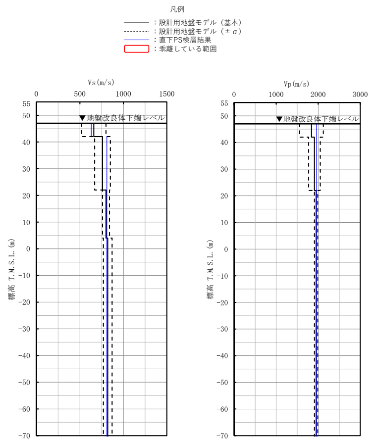
第 3.1-45 図 安全冷却水系冷却塔 A 飛来物防護ネットにおける設計用地盤モデルと直下 PS 検層データとの速度構造の比較結果 (支持地盤)
