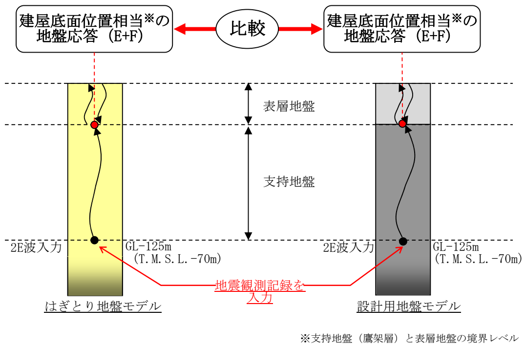
第 4.3-6 図 シミュレーション解析の概要
