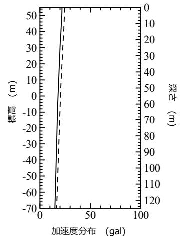
第 4.3-7 図(4) シミュレーション解析結果の 応答スペクトル図 (中央地盤, G.L. -5m) 及び最大加速度分布 (2012 年 5 月 24 日 青森県東方沖の地震)
