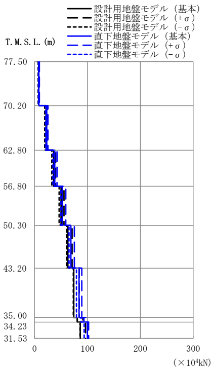
第 2.4.1.1-16 図 最大応答軸力 (鉛直方向 S s -C1 (UD))
