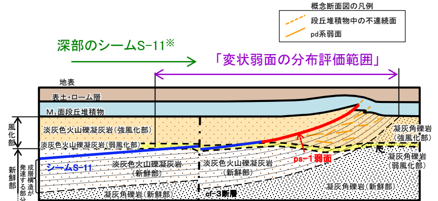
図1 変状弱面の分布評価範囲の概念断面図
