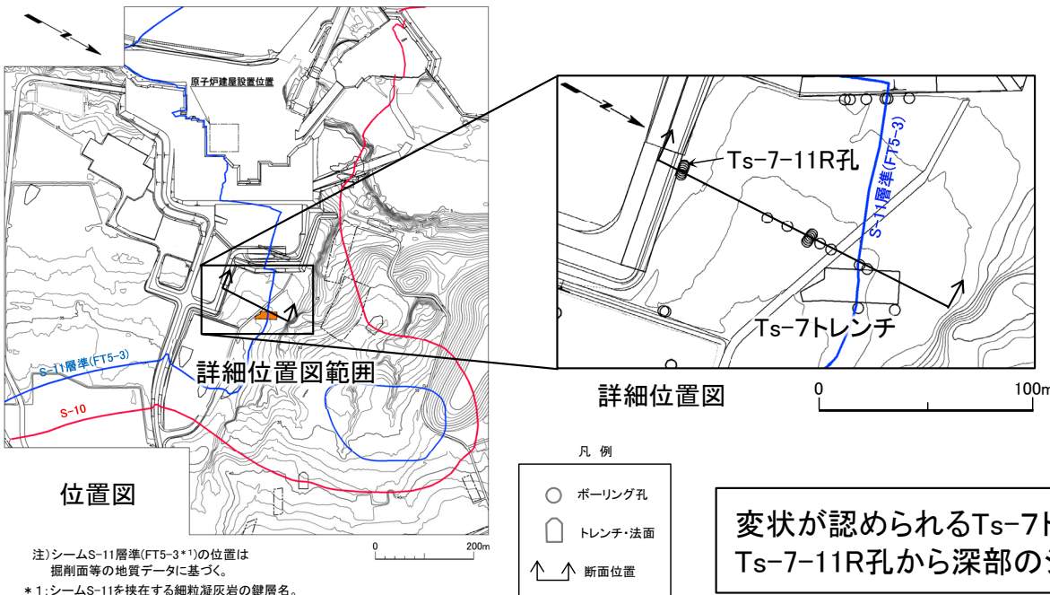
Ts-7トレンチ付近の試料採取位置(断面図)
