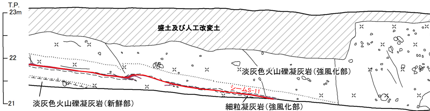
Ts-6a(南)法面
