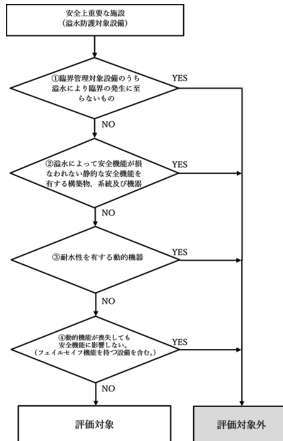
図2-1 溢水評価対象設備の選定フロー
