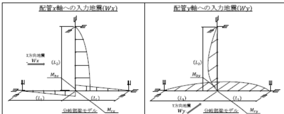
第3.4.2-6図(2/3) 配管（分岐部）モデル
