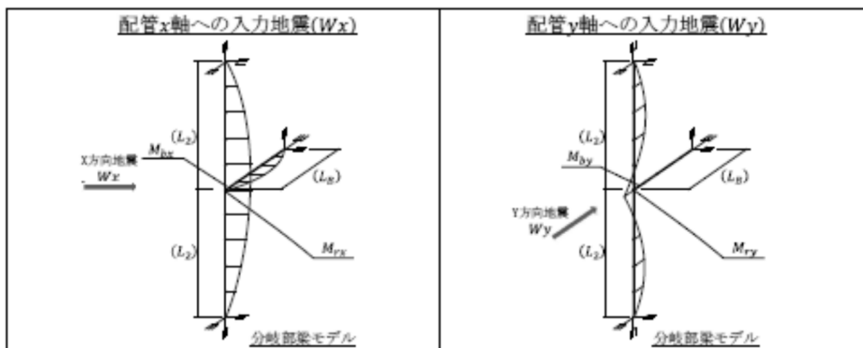
第3.4.2-6図(3/3) 配管（分岐部）モデル
