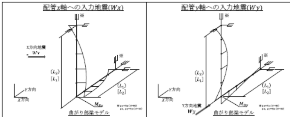
第 3.4.2-4 図(2/2) 配管（曲がり部）モデル
