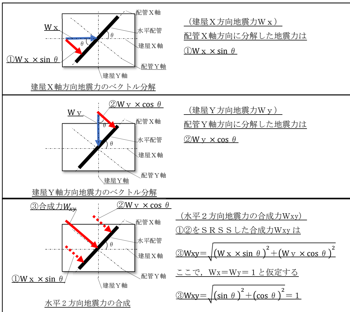
第3.4.2-2図 建屋応答軸と角度を有した配管配置
