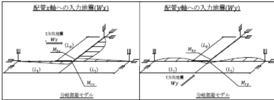
第3.4.2-6図(1/3) 配管（分岐部）モデル
