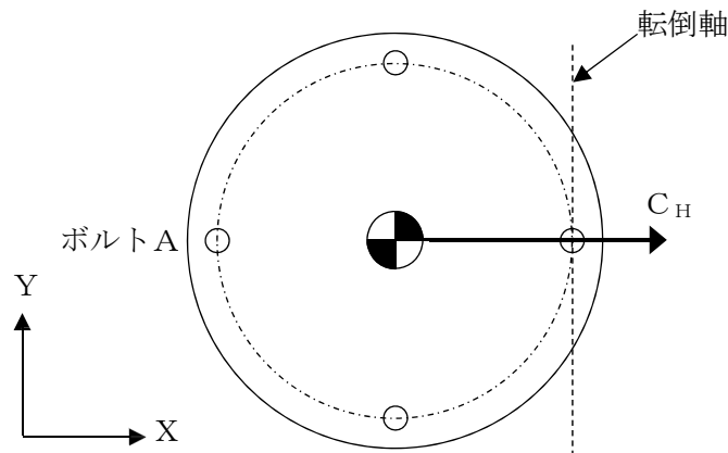
第3.4.5-1図 水平1方向の地震力による応答イメージ
