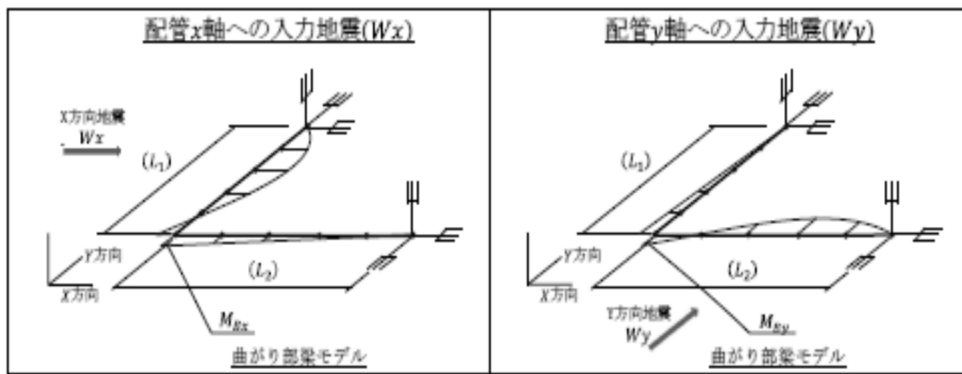
第 3.4.2-4 図(1/2) 配管（曲がり部）モデル
