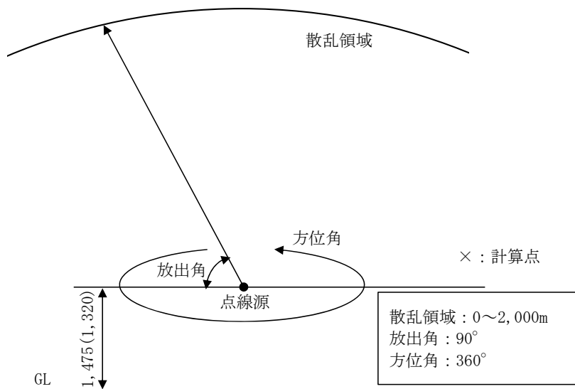
第4図 ANISNによる角度別ガンマ線束の計算モデル
