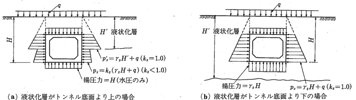
第 5.2.2-1 図 構造物と液状化対象層の位置関係に応じた作用荷重
