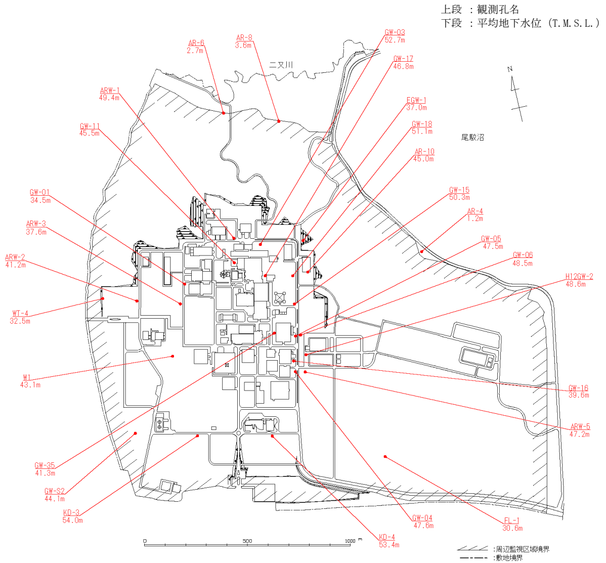
第 2.3-1 図 地下水位観測孔位置及び平均地下水位
