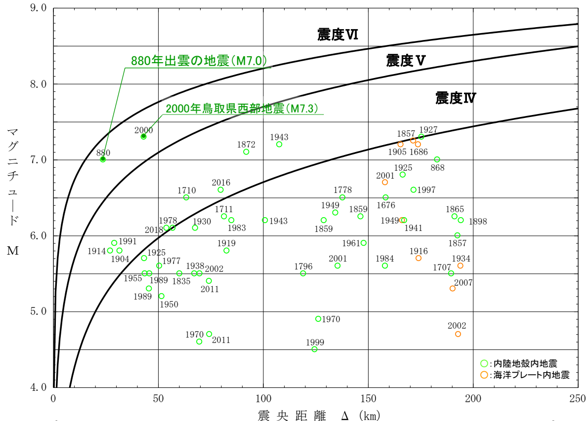
M-Δ 図(～2019年8月)
