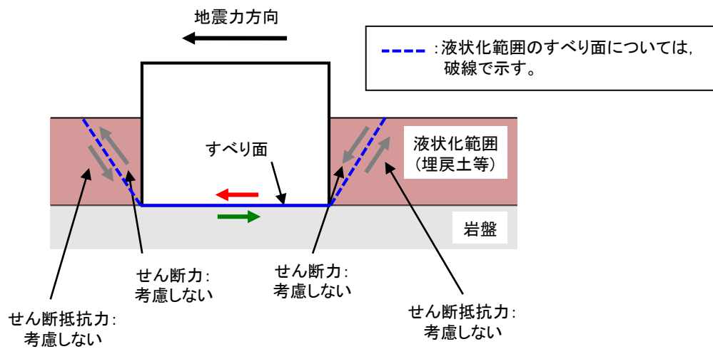
すべり安全率の算定方法(簡便法, 動的解析) イメージ図
