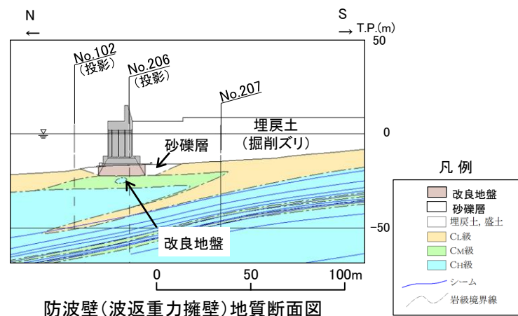
防波壁(波返重力擁壁)地質断面図
