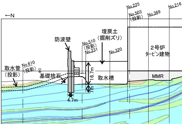
防波壁(多重鋼管杭式擁壁)
