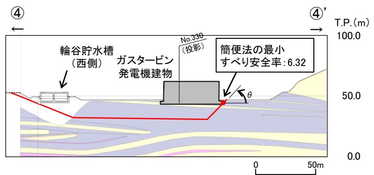
地質断面図(④-④'断面, 岩相)
