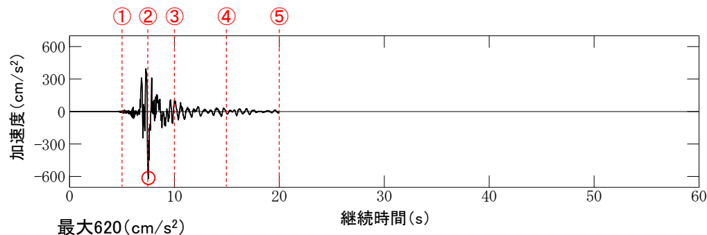
基準地震動 S_s-N1 の時刻歴波形(水平)
