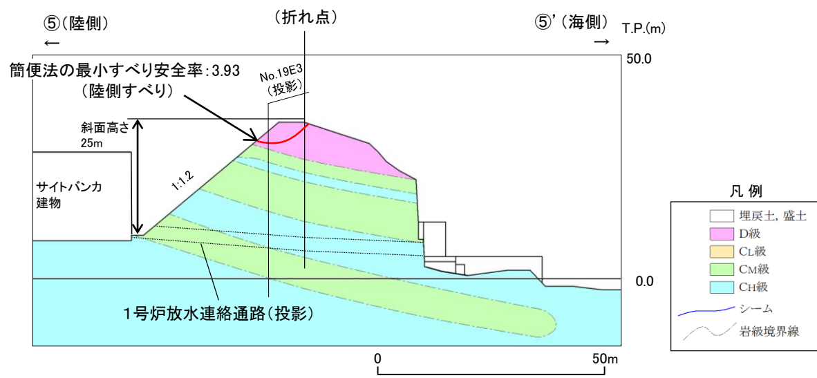
防波壁(東端部)周辺斜面(⑤-⑤'断面, 岩級・シーム)
