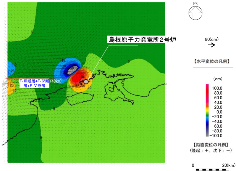
地殻変動解析結果 (F-Ⅲ断層+F-Ⅳ断層+F-Ⅴ断層 上昇最大ケース)
