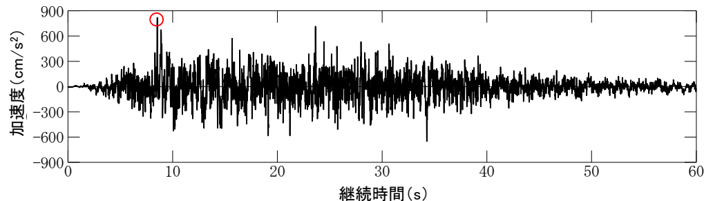
基準地震動Ss-Dの時刻歴波形(水平)
