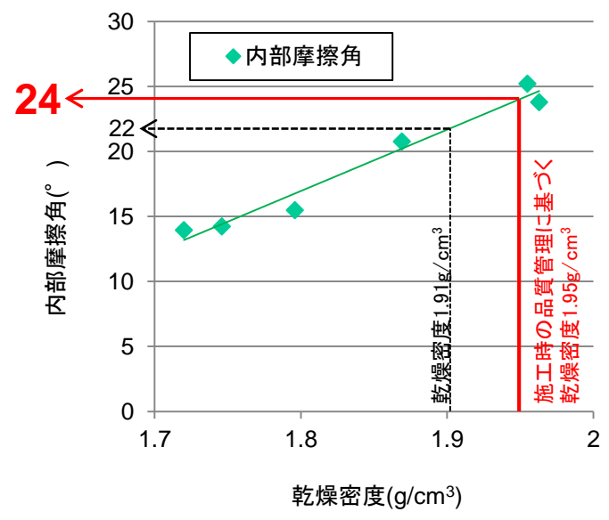
大型三軸圧縮試験結果(2号)
