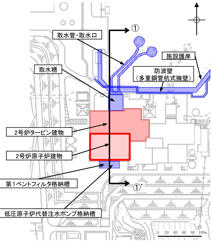
断面位置図
