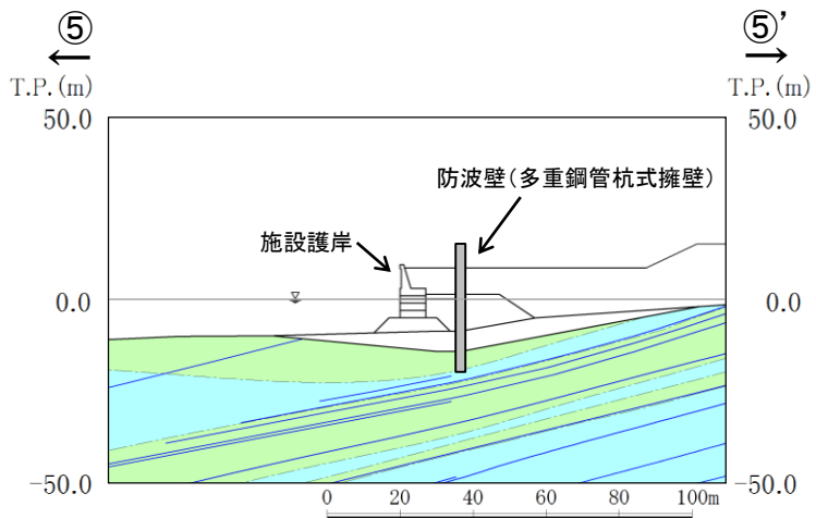
⑤-⑤' 断面図
