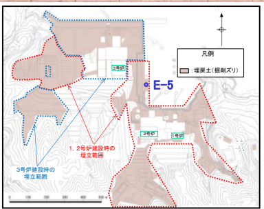
敷地平面図
