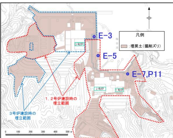
敷地平面図
