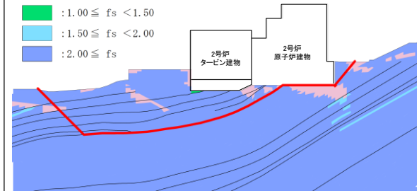
建物影響範囲*2
