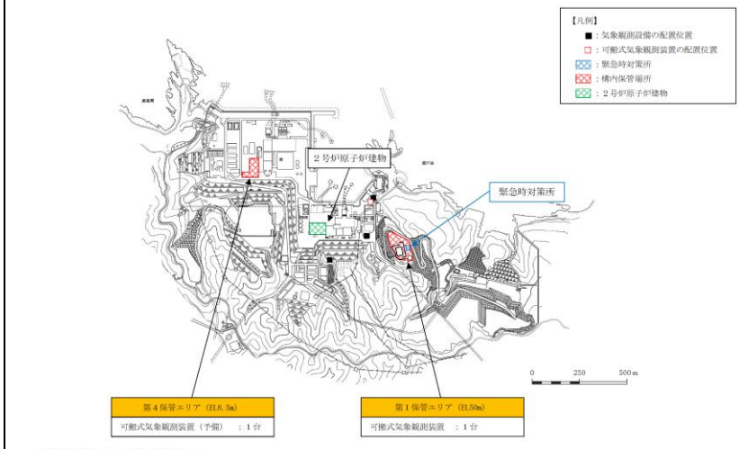
第 1.17-15 図 可搬式気象観測装置の配置位置及び保管場所
