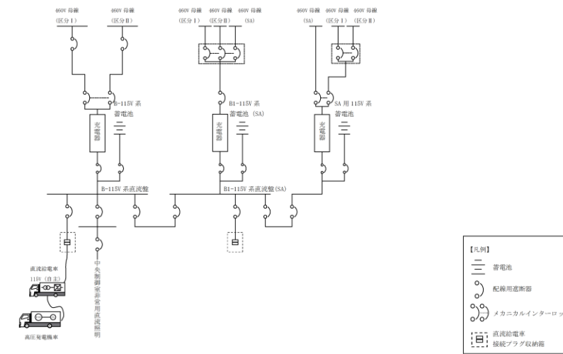
第3図 電源構成図 (直流電源)
