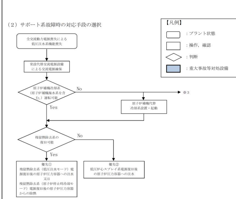
第1.4-33図 重大事故等時の対応手段選択フローチャート (2/3)
