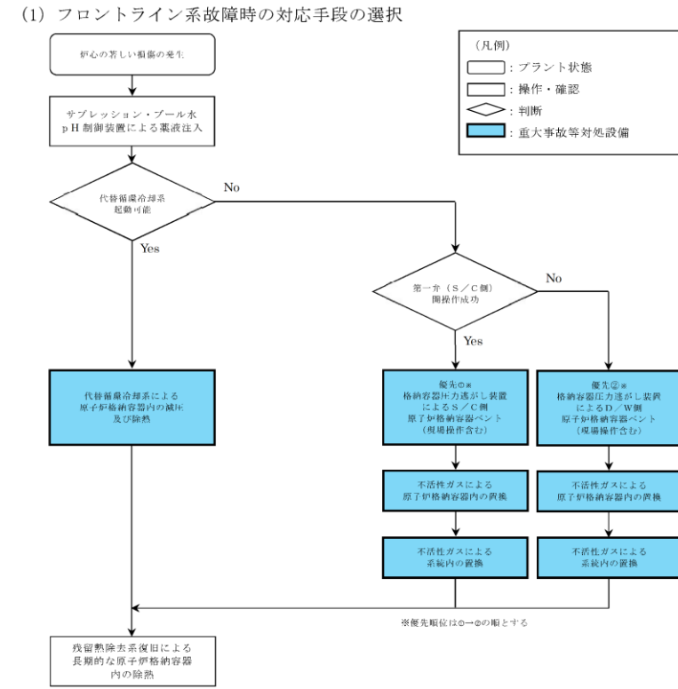
第 1.7-20 図 重大事故等時の対応手段選択フローチャート
