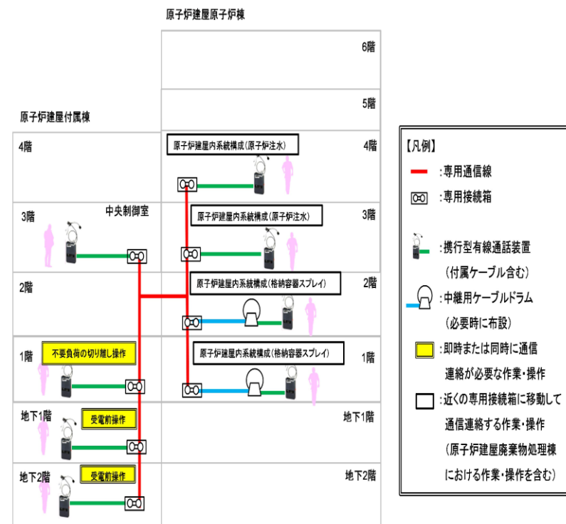
図62-6-7 携帯型音声呼出電話機を用いた通信連絡の概要 (重大事故シーケンス 全交流動力電源喪失時 (7号炉) の例)
