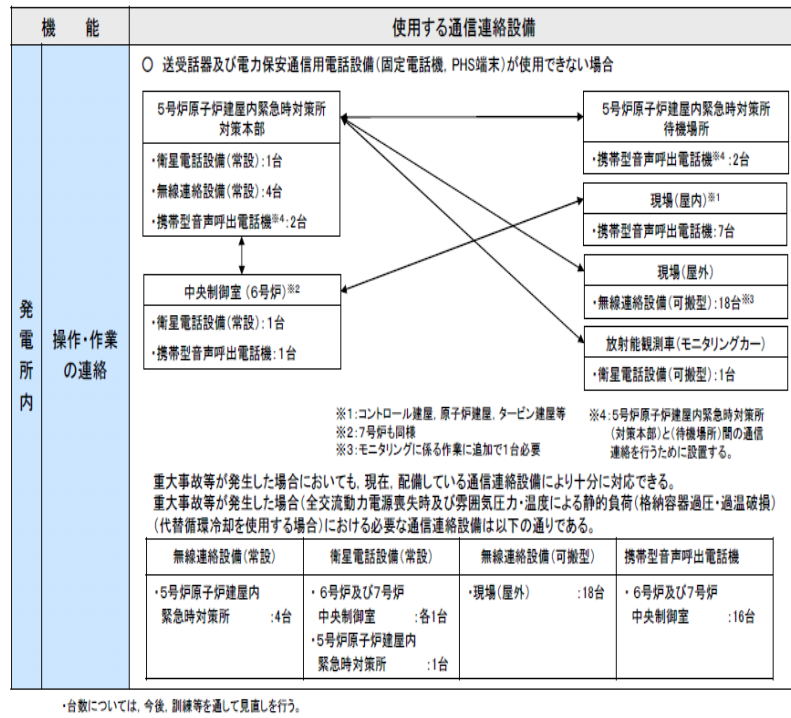
図62-6-3 機能ごとに必要な通信連絡設備(発電所内) (3/4)
