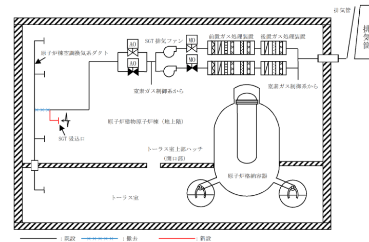
図1 SGT系統概要図
