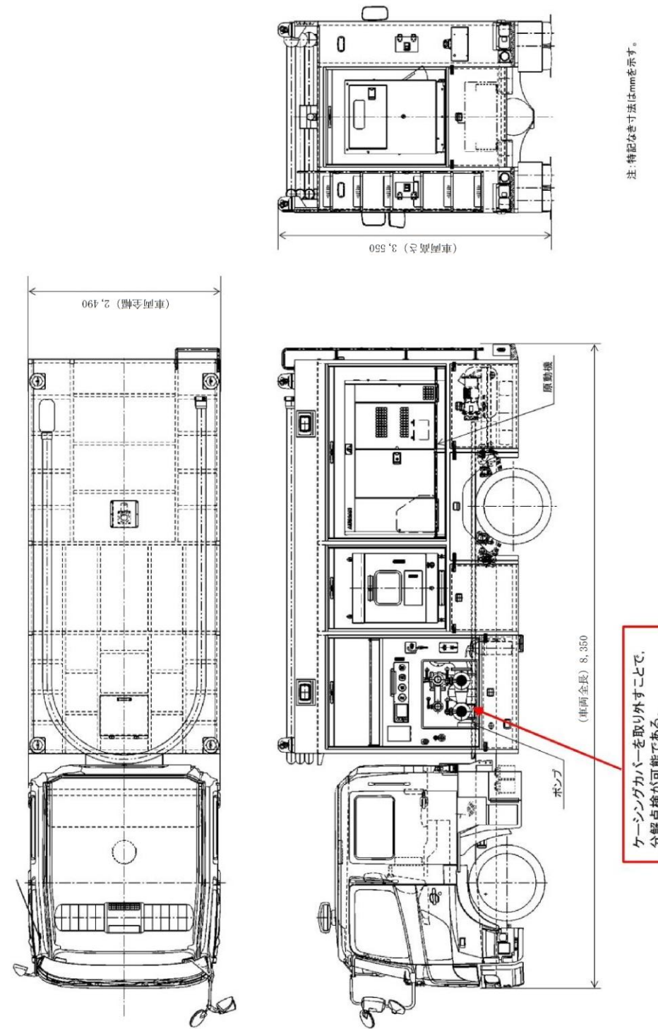
図2 大量送水車構造図
