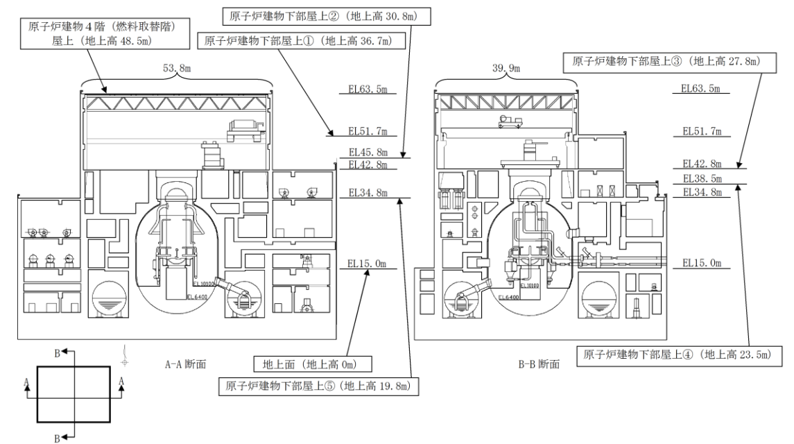
図 5-4 原子炉建物断面図
