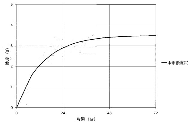
図 2-7 原子炉建屋（原子炉建屋オペレーティングフロア）水素濃度の時間変化
