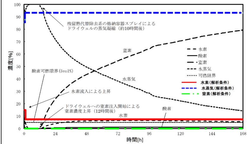
図 2.2.2-13 D/W 内ガス条件 (RHAR ケース)
