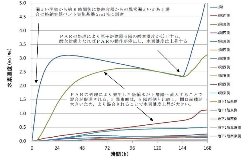
第 2.1.4.2-3 図 ケース 2 水素濃度の時間変化 (原子炉建屋原子炉棟全域)
