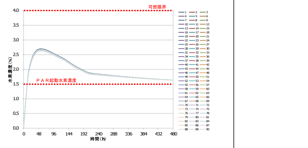
図 2.2.2-16 原子炉建物原子炉棟 4 階の全サブボリュームの水素濃度の時間変化 (設計条件, ベント無し)
