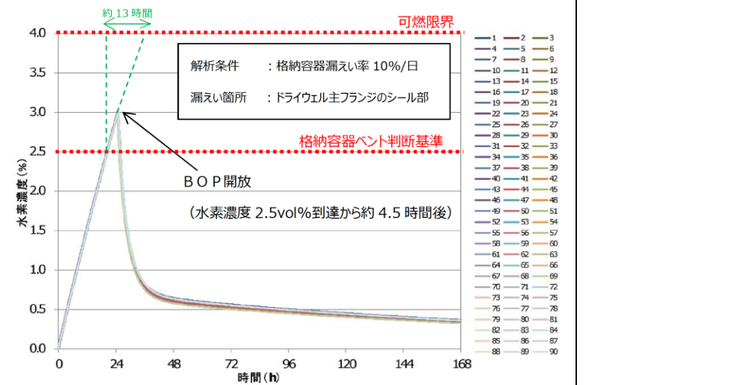
図11 原子炉建物燃料取替階ブローアウトパネル開放による水素濃度の時間変化 (PAR及び格納容器ベント不作動時)
