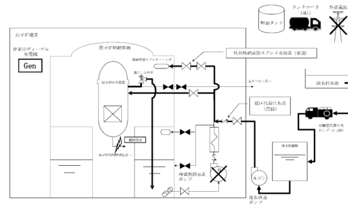
第 2.6.2 図 「LOCA 時注水機能喪失」の重大事故等対策の概略系統図 (2/3) (原子炉注水及び原子炉格納容器冷却)
