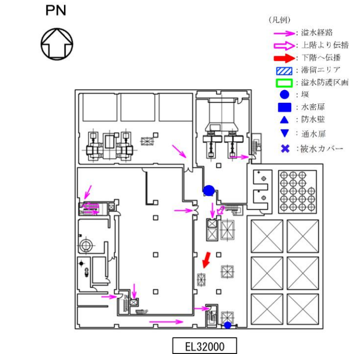
図 2-31 廃棄物処理建物 4階 溢水防護対策設備設置箇所
