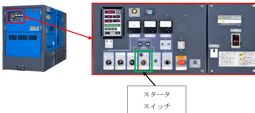
第2.3-2図 緊急時対策所用発電機から受電時の操作（夜間時）
