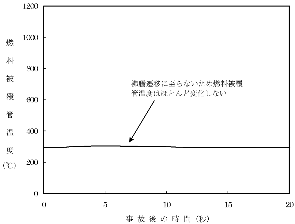
図 6-4 R/B における内部溢水による事象変化 (燃料被覆管温度) (主蒸気隔離弁の誤閉止)
