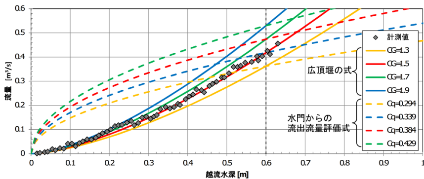
図 3-5 通水扉越流水深と流量の関係
