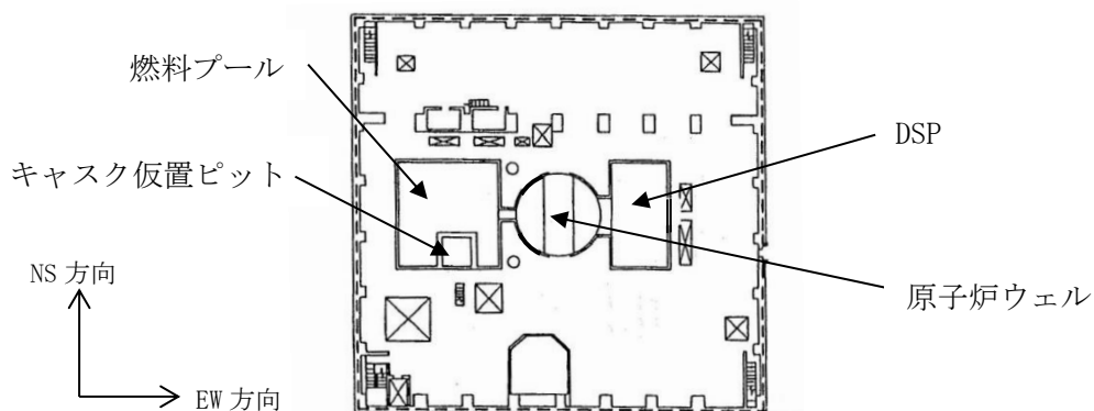
図 1 原子炉建物 4 階の機器配置図
