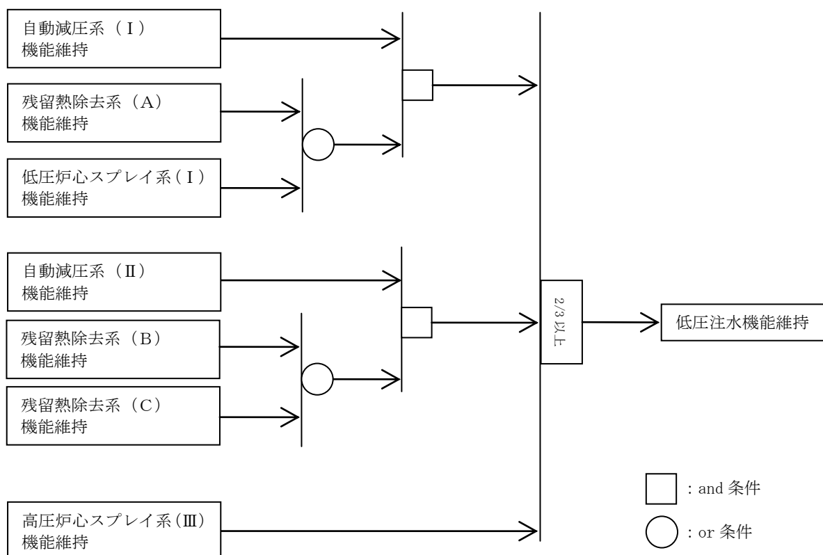
図3 安全機能判定フロー(低圧注水機能)
