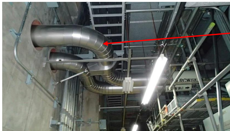
図2 溢水源となり得る機器の確認例 (R-B2F-05N)
