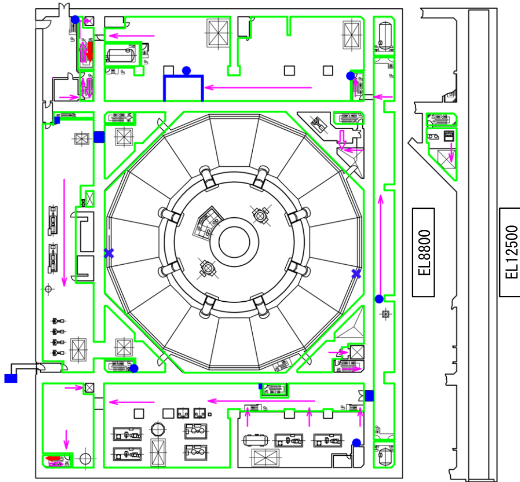
図 2-19 原子炉建物地下 1 階 溢水防護対策設備設置箇所
