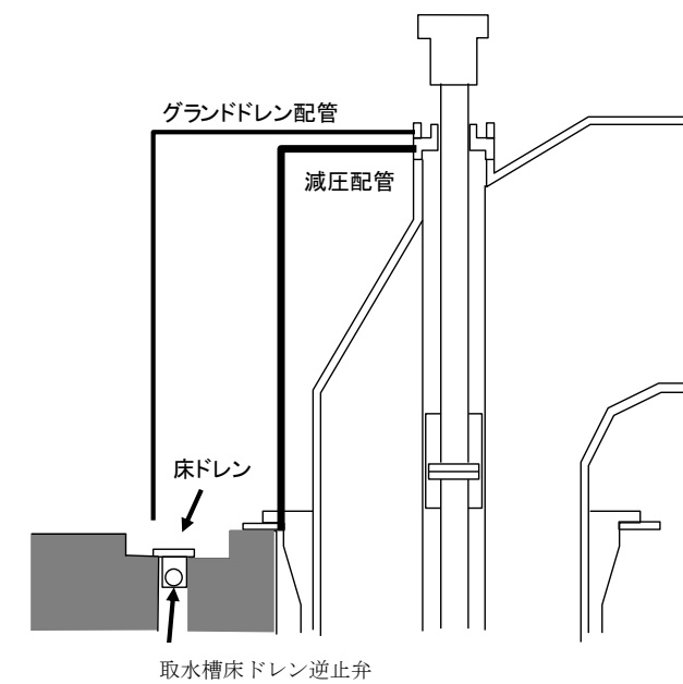
第2.3-5図 循環水ポンプのグランド dren 等配管ルート
