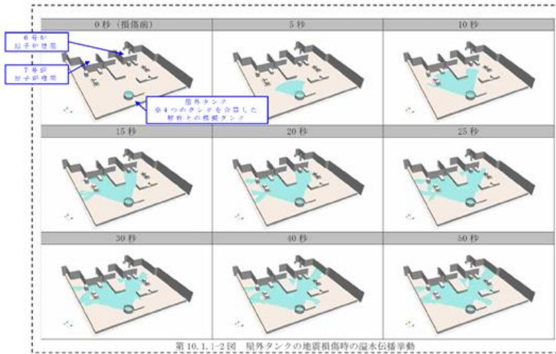
第10.1.1-2図 屋外タンクの地震相傷時の溢水伝播挙動
