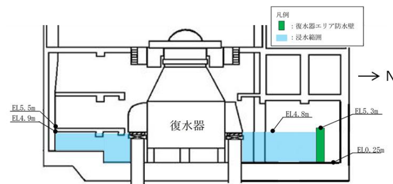
(A-A 断面)
