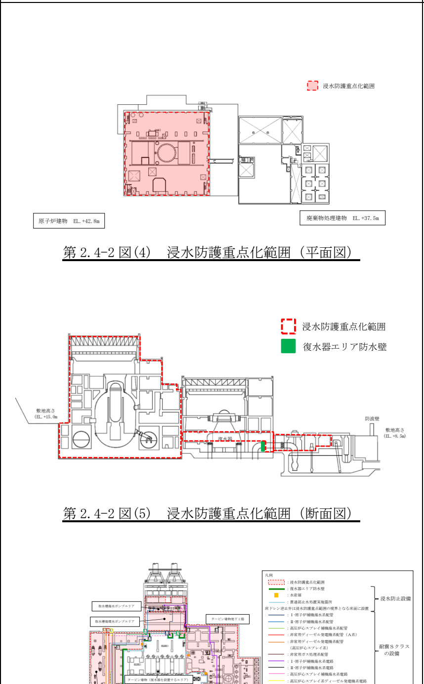
第2.4-3図 タービン建物地下1階の復水器エリア防水壁等の浸水防護重点化範囲と耐震Sクラスの設備の位置
