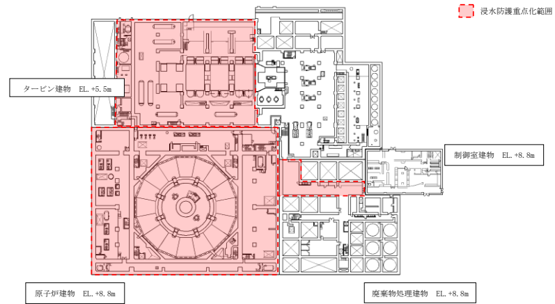
第 2.4-2 図(1) 浸水防護重点化範囲(平面図)
