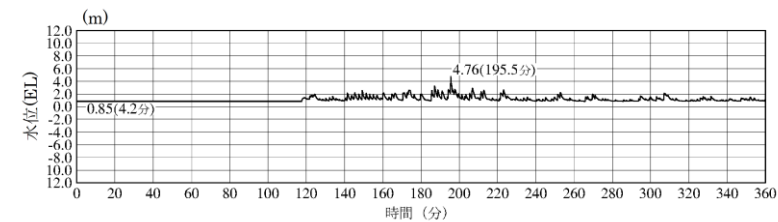
第 2.2-26 図 1号炉放水槽での入力津波の時刻歴波形（上昇側） （入力津波1：防波堤有り）
