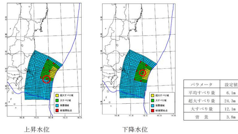
第2図 東海第二発電所の基準津波の波源
