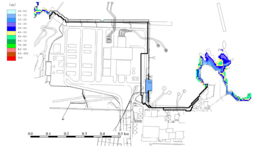
第1.3-2 図 基準津波による遡上波の最大浸水深分布 (基準津波1：防波堤無し)
