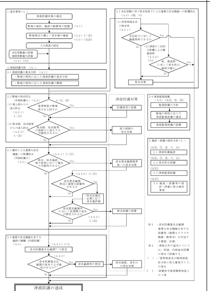
第1図 耐津波設計の基本フロー
