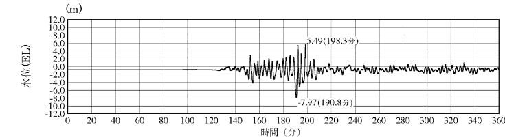
※最大水位下降量-7.97m-地殻変動量0.34m≒EL. -8.4m 2号炉取水槽 (入力津波6, 防波堤無し) ※下降側 ポンプ運転時
