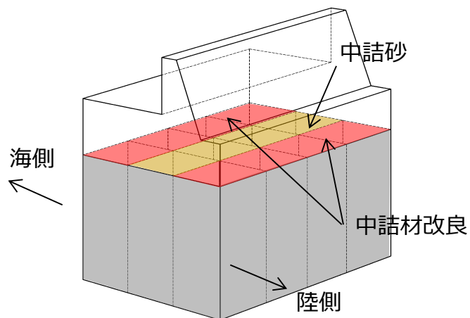
ケースン（輪谷部）構造概念図
