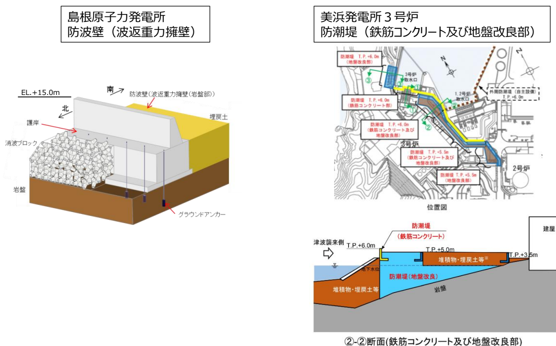
②-②断面(鉄筋コンクリート及び地盤改良部)
