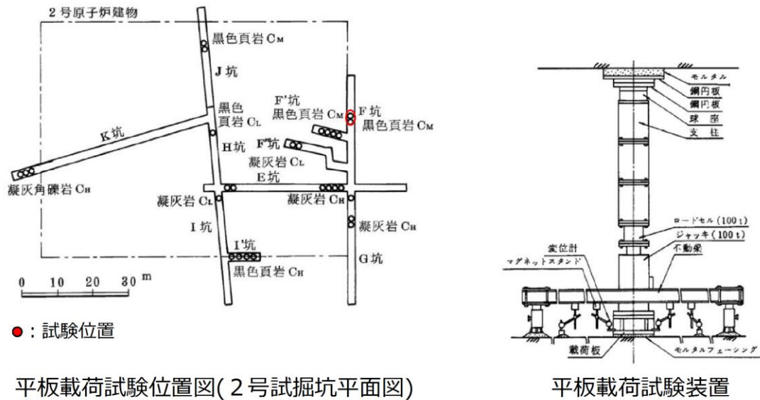
第6-31図 防波壁（逆T擁壁）平板载荷試験概要
