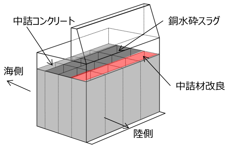
ケースン（改良地盤部）構造概念図
