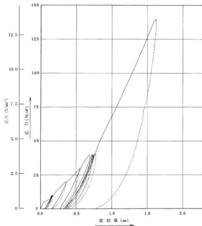
第6-32図 防波壁（逆T擁壁）平板载荷試験結果
