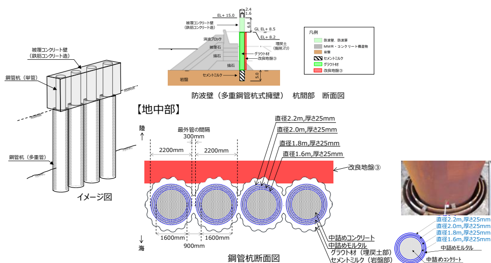
第5-2図 防波壁（多重鋼管杭式擁壁）の構造概要図
