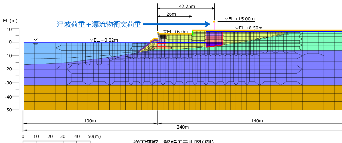
逆T擁壁 解析モデル図(例)
