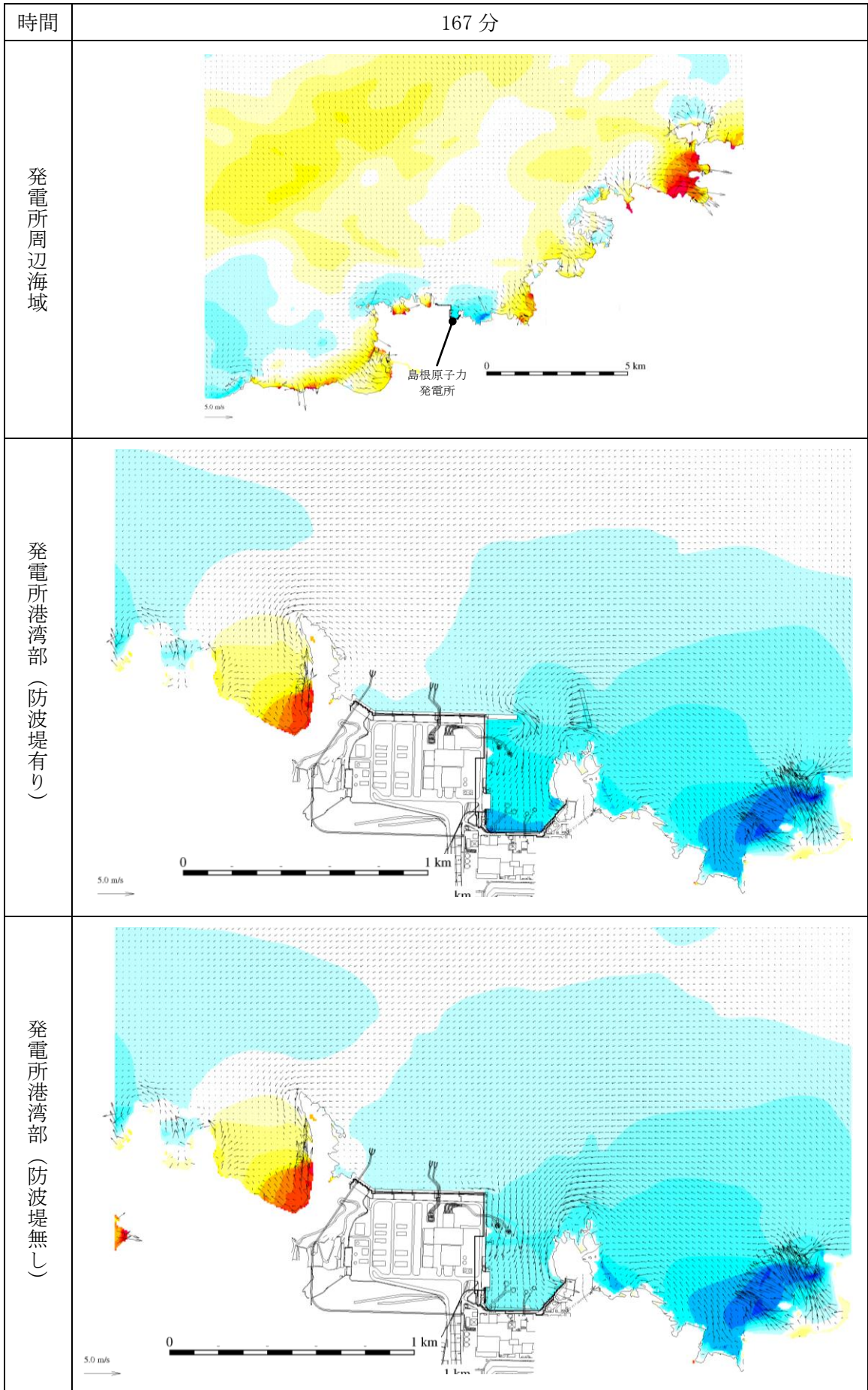
第 1 図(135) 基準津波 1 の水位変動・流向ベクトル
