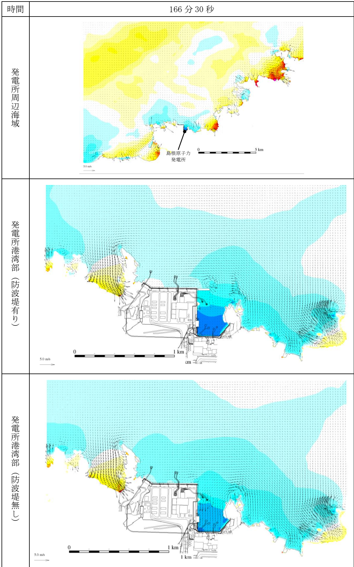
第 1 図 (134) 基準津波 1 の水位変動・流向ベクトル
