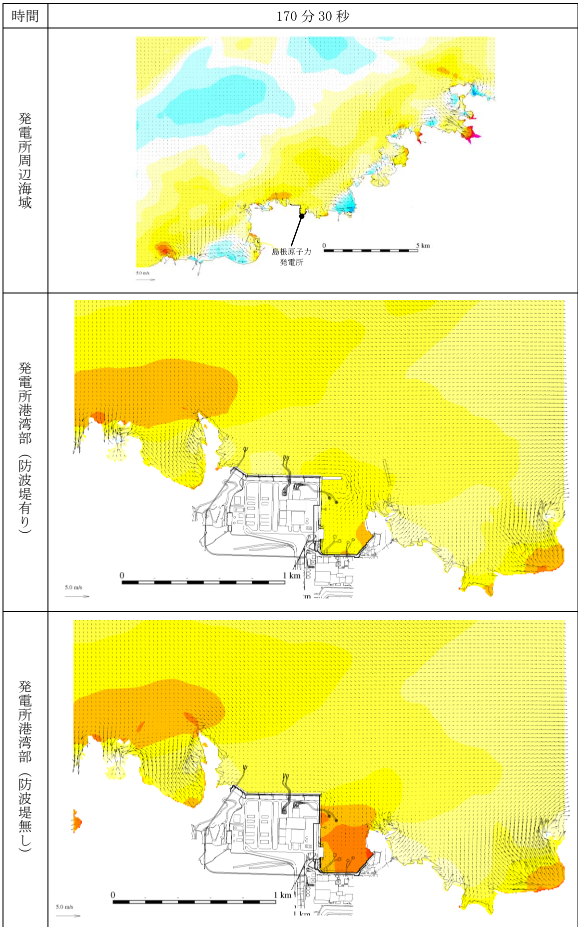
第 1 図(142) 基準津波 1 の水位変動・流向ベクトル
