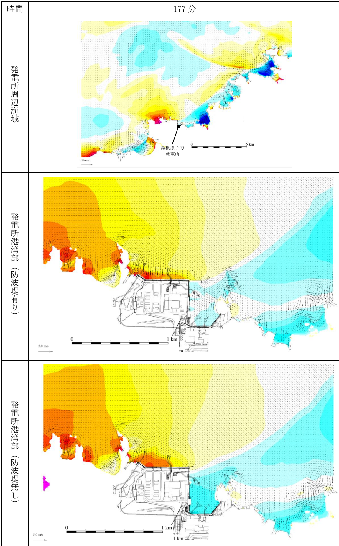
第 1 図(155) 基準津波 1 の水位変動・流向ベクトル
