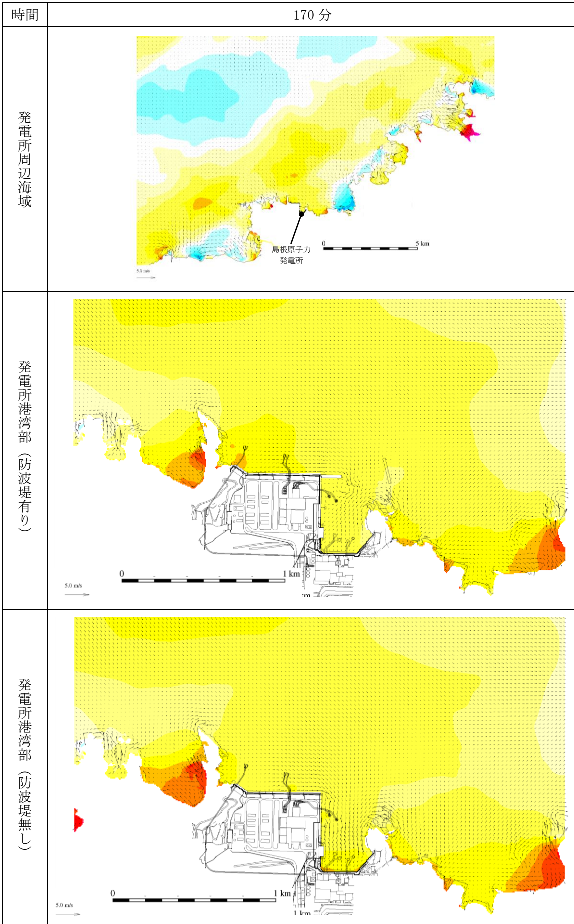
第 1 図(141) 基準津波 1 の水位変動・流向ベクトル
