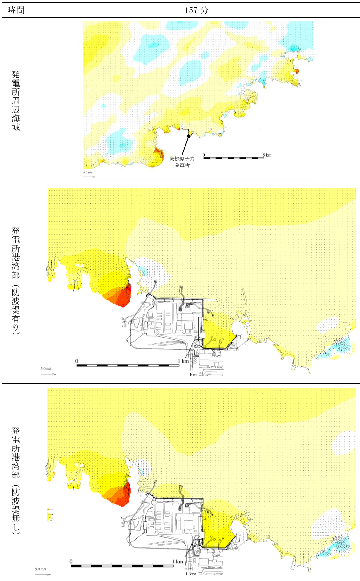
第 1 図(115) 基準津波 1 の水位変動・流向ベクトル
