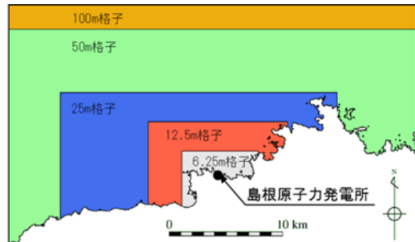
計算格子分割
