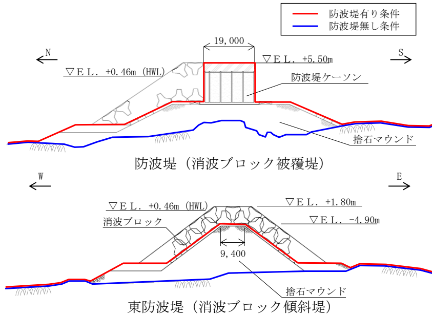
図5-2 防波堤断面図
