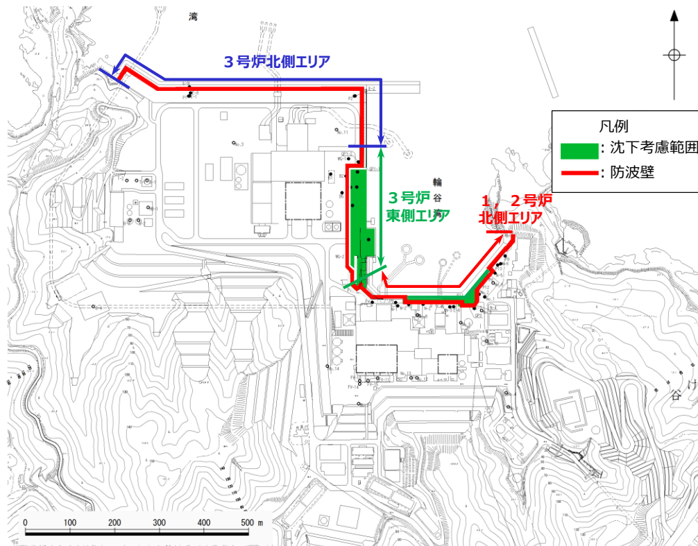
図3-8 敷地平面図
