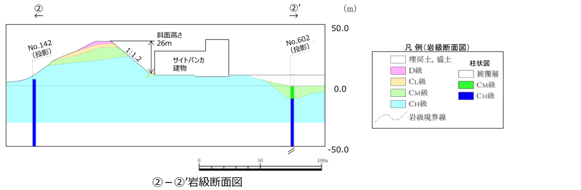
図 2 - 9 (2) 防波壁 (東端部) 地質断面図・岩級断面図 ②-②' 断面
