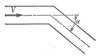
図7 屈折角 (発電水力演習p.88)
