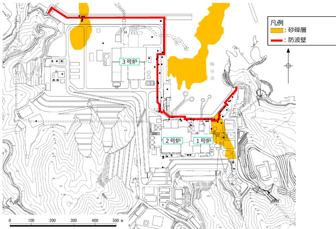
图 3-4 (3) 砂礫層分布图
